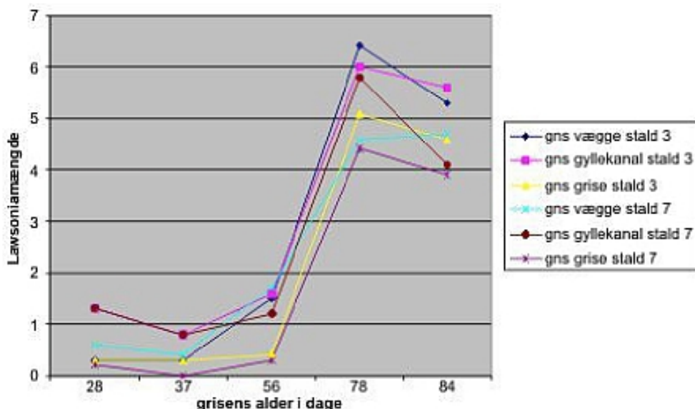
Figur 3. Gennemsnitlig mængde af påviste Lawsoniabakterier i grise og prøver udtaget på vægge og i gyllekanaler i to smågrisestalde i besætning 2 (C2). Mængden af bakterier er vist på en skala fra 0 til 7. Værdien 1 svarer ca. til 104 bakterier/g gødning. Ved værdier under 1 er mængdebestemmelsen usikker. Da der er tale om en eksperimentel PCR til forskningsbrug er der anvendt en relativ skala som skal tages med et vist forbehold. Billede nr. 2296
