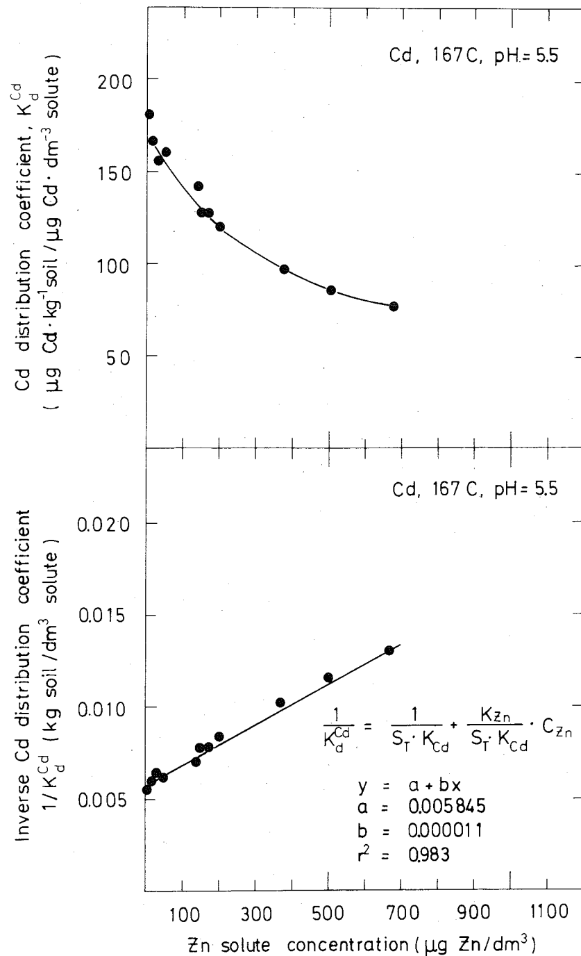
Figur 8.6 K_d -værdien for cadmium på en sandjord som funktion af tilstedeværelsen af zink i opløsningen 6 .
