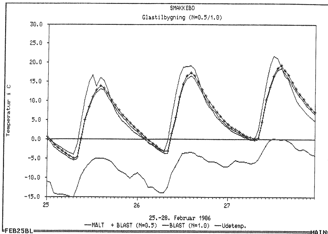
Figur 4.3-16. Luftsiftets indflydelse på de beregnede værdier med BLAST, for et naturligt luftskifte på henholdsvis en halv og én gang pr. time.
