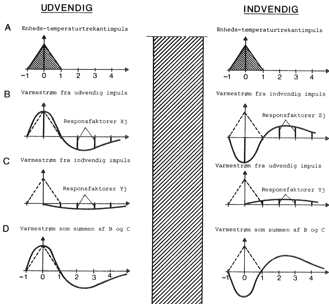
Figur 2.2-9. Skematisk illustration af varmestrømme ved hjælp af superpositionsprincippet (varmestrømmen er fortegnet).
