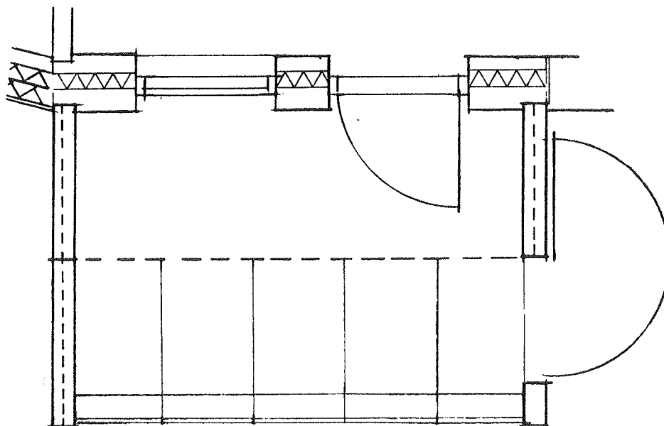
Figur 4.3-13. Plan over glastilbygningen.
