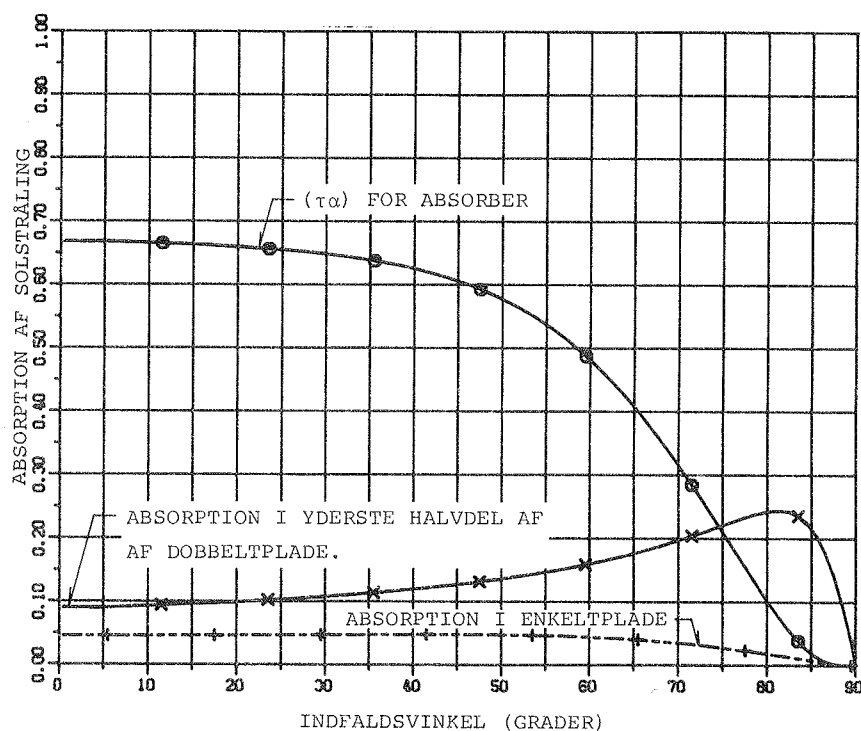
Fig. Al.7.5 Resulterende transmissions-absorptionsprodukt for absorber og absorption i dæklag. Dæklagskonstruktion af plexiglas dobbelt- og enkeltplade . Solindfald ved forskellige solhøjder, azimut = 0 . Vandrette ribber i dobbeltplade.
