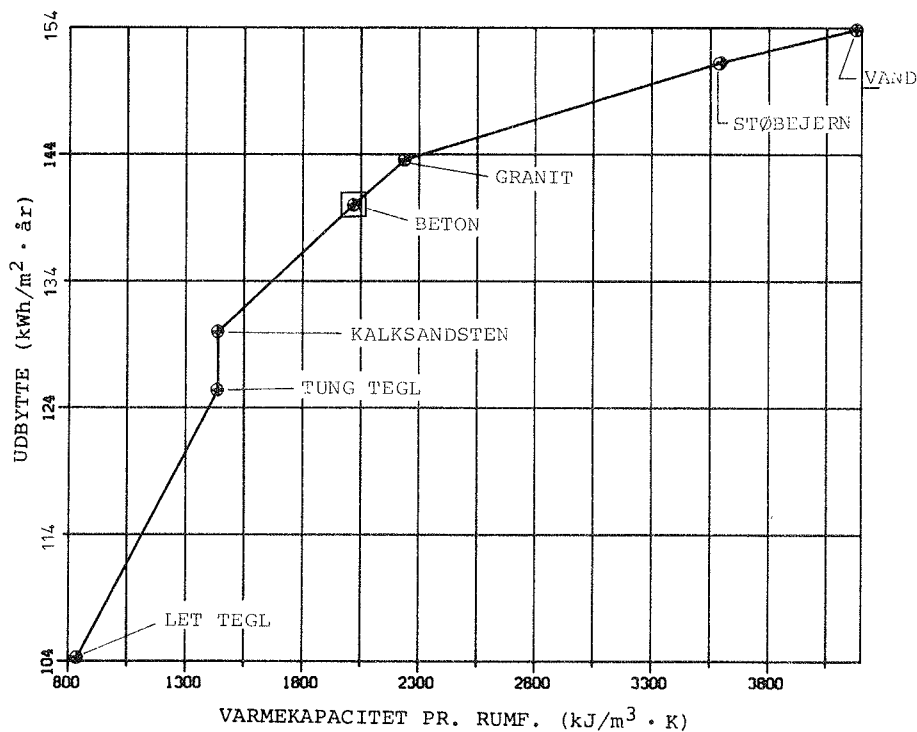
Fig. 2.3.7 Udbytte af solvæg med forskellige typer varmelager. Varmelagerets tykkelse er 0,228 mm. Referencesolvæggen er markeret med □.
