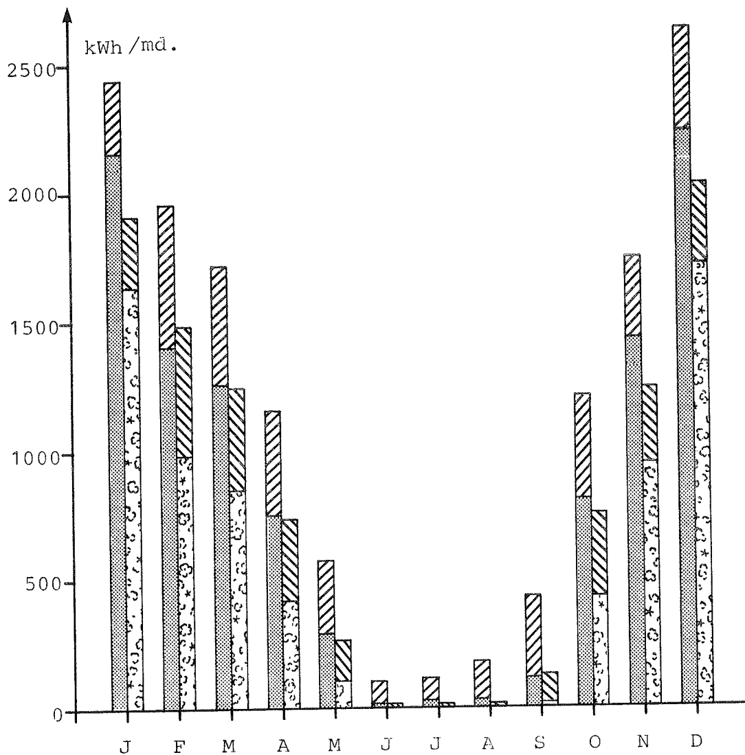
Fig. 2.2.8 Opvarmningsbehov på månedsbasis i hus med og uden brugsvarme og med og uden 27 m 2 mobilisoleret solvæg (som i forsøg, dog betonlager). Hustype: BR-82 hus, mobil natisolering for vinduer, middeltungt hus, 9 m 2 vinduesareal mod syd.
