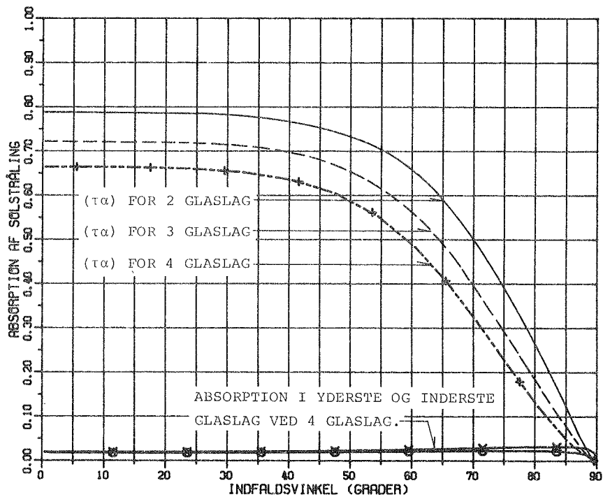
Fig. Al.7.10 Resulterende transmissions-absorptionsprodukt for solvæg med dæklagskonstruktion af 2-4 lag jernfrit glas ved forskellige indfaldsvinkler og absorption i glaslaget.
