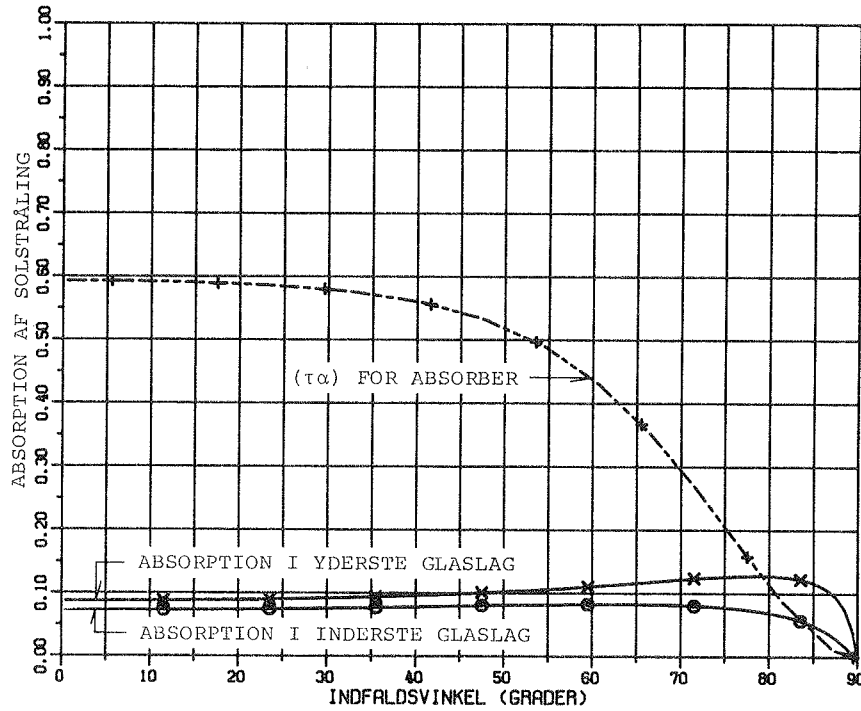
Fig. Al.7.9 Resulterende transmissions-absorptionsprodukt for absorber og absorption i dæklag med dæklagskonstruktion af 3 lag almindeligt glas. Solindfald ved forskellige indfaldsvinkler.
