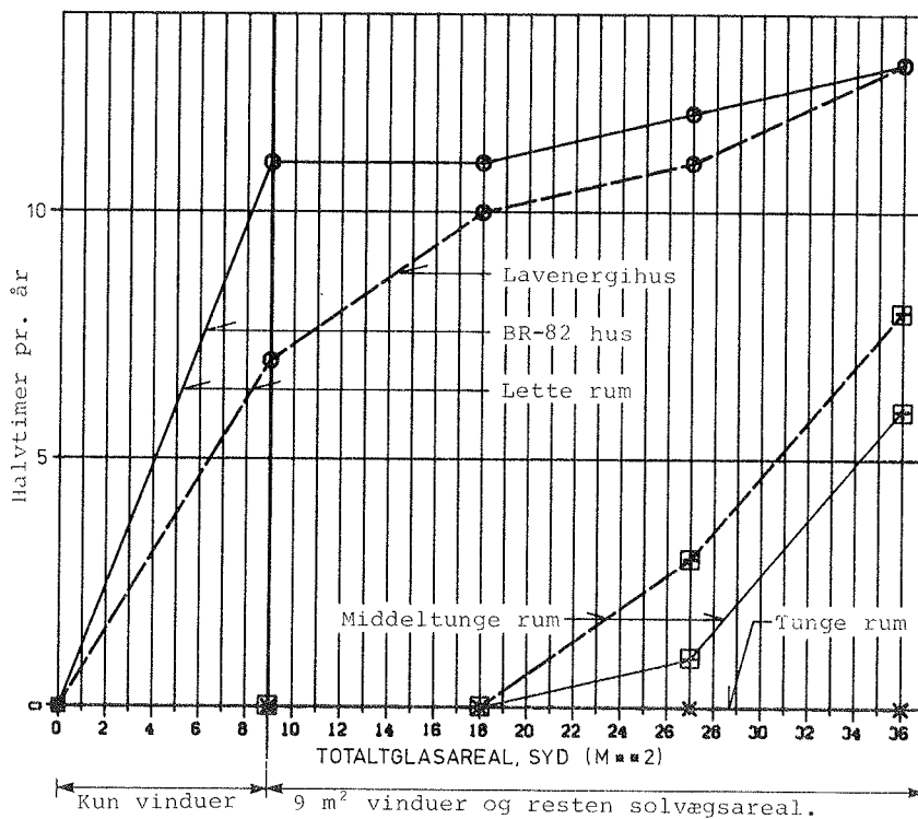
Fig. 2.2.6 Antal halvtimer med rumlufttemperaturer over 25^{\circ}\text{C} i månederne oktober til april (incl.). Mobiliseret solvæg som i forsøg dog betonlager. Ingen mobil natisolering for vinduer. Normal brugsvarme fra el og personer.
