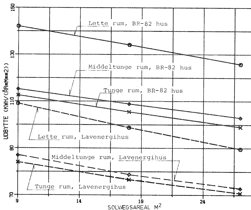
Fig. 2.2.4 Udbytte af mobilisoleret solvæg ved varierende tyngde og glasareal mod syd. Solvæg som i forsøg dog betonlager. Ingen mobil natisolering for vinduer. Normal brugsvarme fra el og personer.
