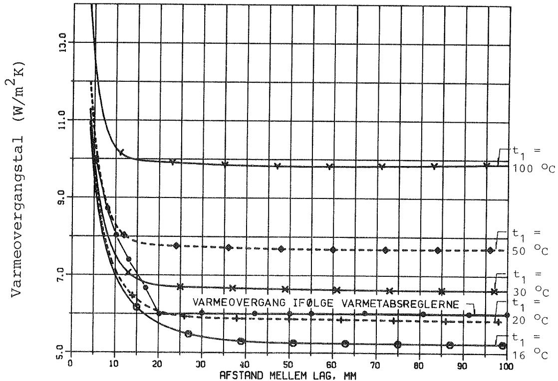
Fig. Al.2.4 Varmeovergangstallet mellem to lodrette planparallelle overflader med emissionskoefficienten \epsilon_h = 0,95 . Overfladernes temperaturer er t_2 = 15^\circ\text{C} og t_1 som vist.
