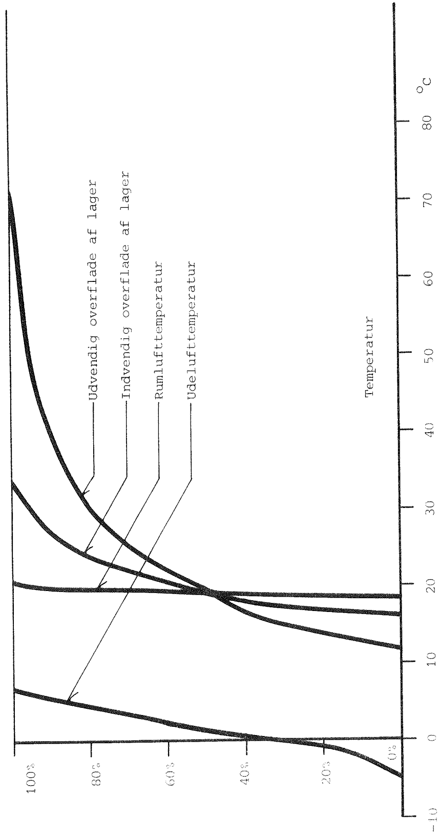
Fig. 4.1.12 Kumuleret fordeling af rumluft- og udelufttemperatur samt udvendig og indvendig overfladetemperatur for solvæg med selektiv absorberoverflade (væg A) i perioden 24/2-12/3-83.
