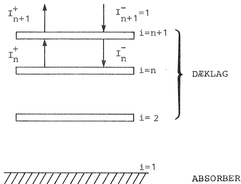
Fig. Al.6.1 Dæklagsystem med tilhørende størrelser af transmitteret stråling.
