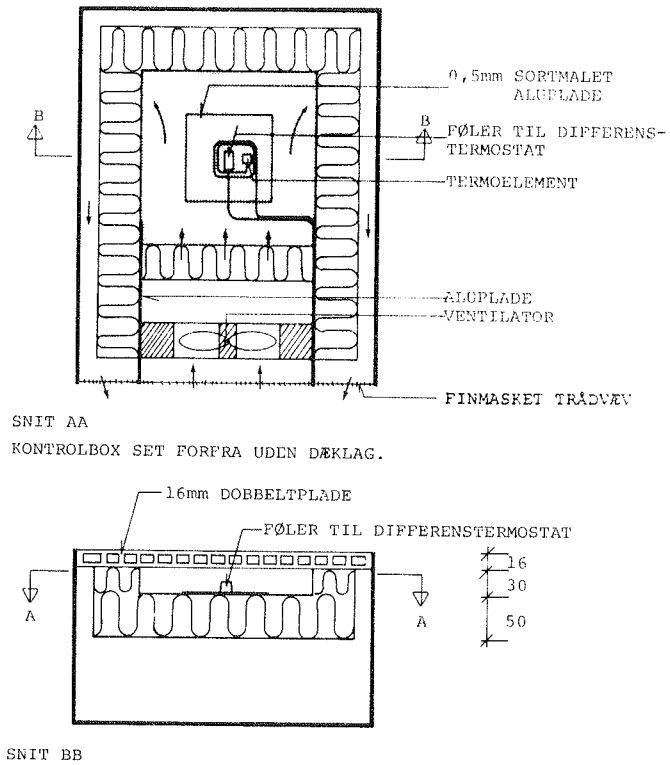
Fig. 3.1.12 Kontrolbox.
