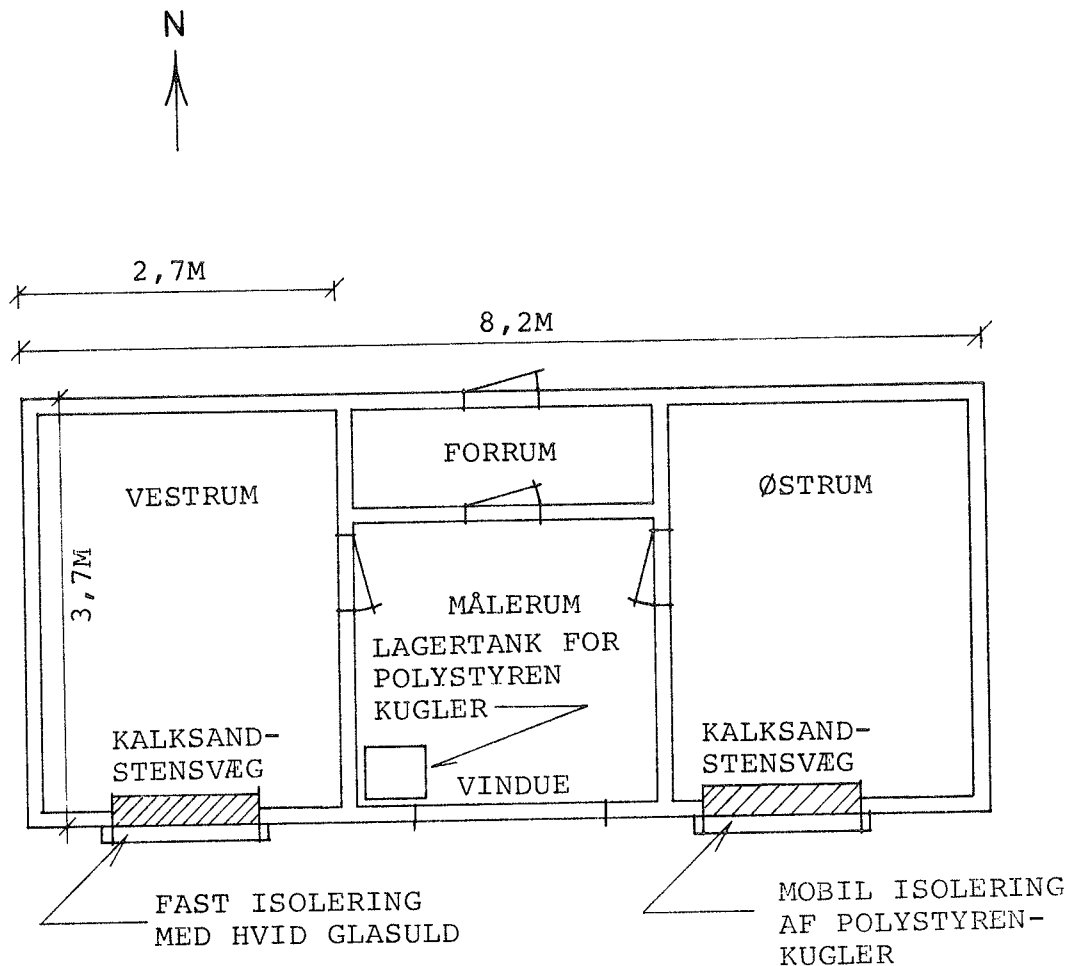
Fig. 3.1.1 Oversigtsplan af forsøgshus med solvægge.
