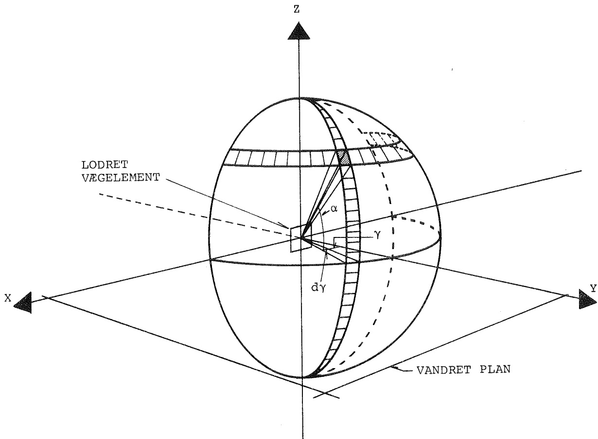
Fig. A1.7.1 Opdeling af halvkugle ved integration.
