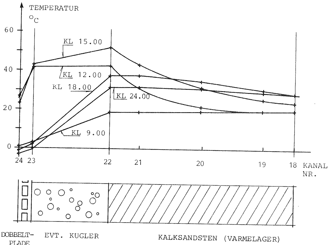
Fig. 4.1.1 Temperaturforløb gennem solvæg med mobil isolering, 24/2 1979.
