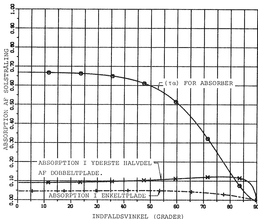
Fig. Al.7.4 Resulterende transmissions-absorptionsprodukt for absorber og absorption i dæklag. Dæklagskonstruktion af plexiglas dobbelt- og enkeltplade . Solindfald ved forskellige azimutvinkler, solhøjde = 0 . Vandrette ribber i dobbeltplade.
