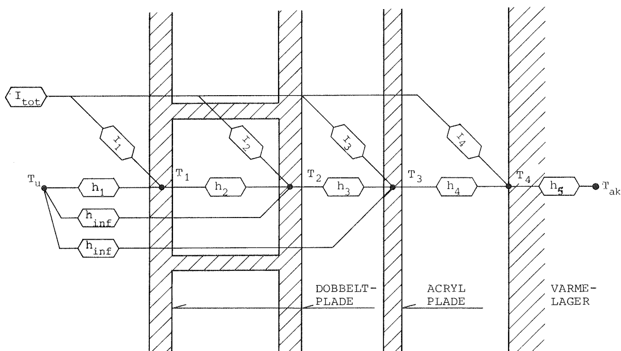
Fig. Al.8.1 Opdeling i knudepunkter af dæklag i solvæg med mobil isolering.
