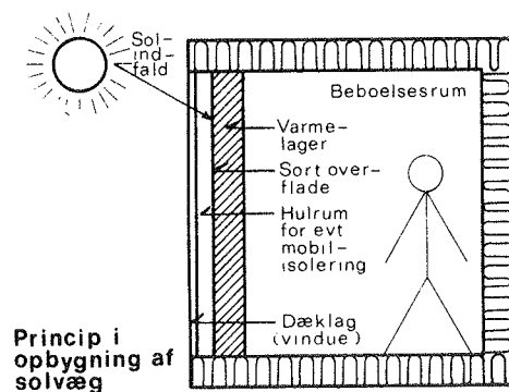
Fig. 1.1.1 Princippet i en solvæg
