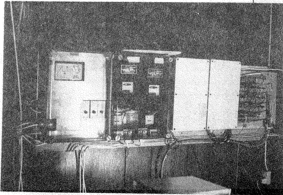
Fig. 3.2.3 Måle- og kontroludstyr. Fra venstre kontrolbox, registrering af injektorventilatorer, primær og sekundær temperaturreference samt fordelelpanel.
