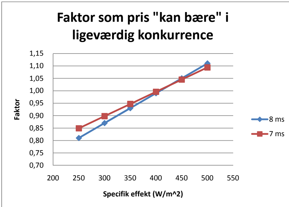
Figur 23 Et delresultat af den udviklede prisenregner er hvor meget merpris en større generator til den samme mølle (eller omvendt), en vindmølle kan bære. Det ses at hvis man øger effekten med 25% fra 400 til 500 W/m 2 , kan dette "bære" en merpris på ca. 10% - mindre ved ringere vindforhold og mere ved bedre vindforhold.
