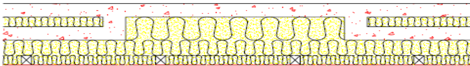
Figur 12. Eksempel på indvendig efterisolering med friholdt skelet – vandret snit i hulmur med radiatorniche, som findes i mange ældre muremesterhuse, men ikke i det aktuelle hus.
