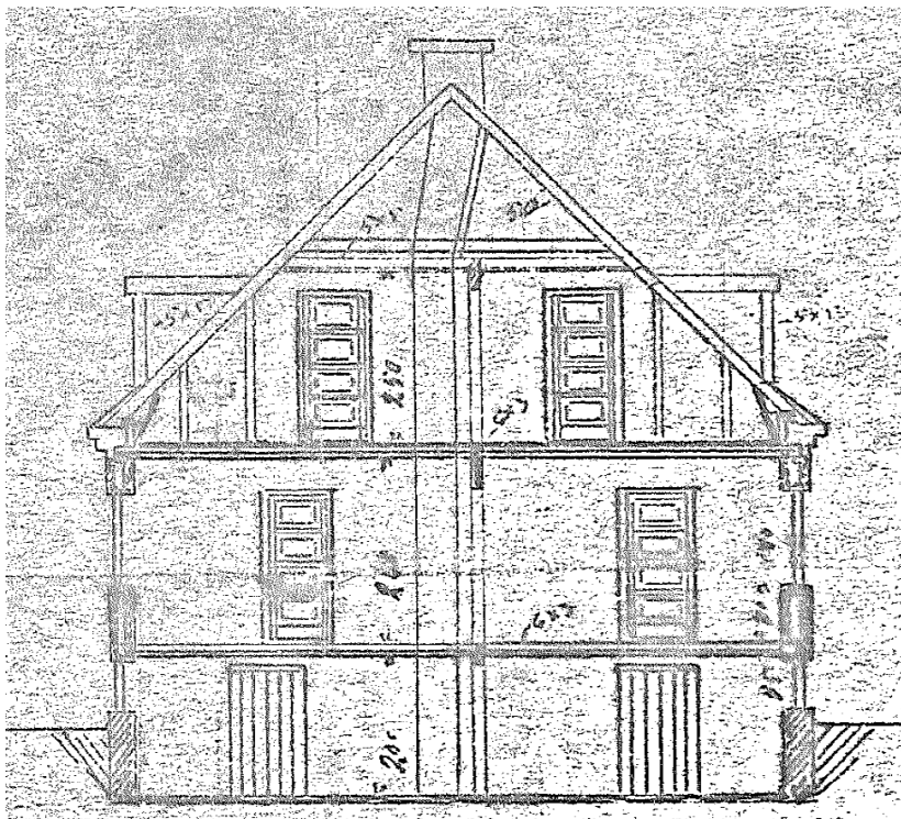
Figur 3. Oprindeligt snit.
