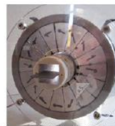
Figura 2: El diseño de de Halbach por Engelbrecht et al. (2007). Puede verse también el regenerador con una placa magnetocalórica
