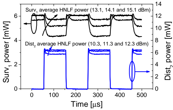
(b) Post-equalizer
