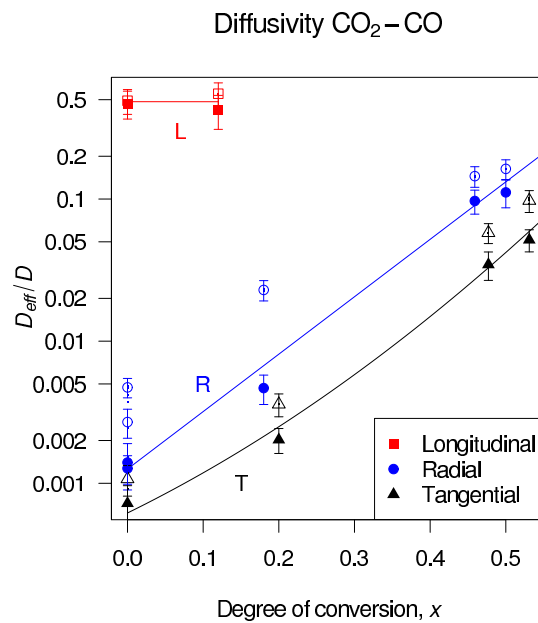
(b) Gas pair CO 2 -CO. □ ○ △: CO 2 ; ■ ● ▲: CO.
