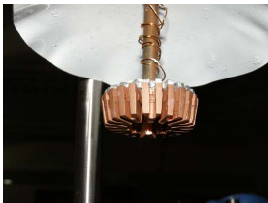
Figur 4 Eksperimentel opstilling af en Cluster enhed hvor lysdioderne er monteret på en kobberroset.
