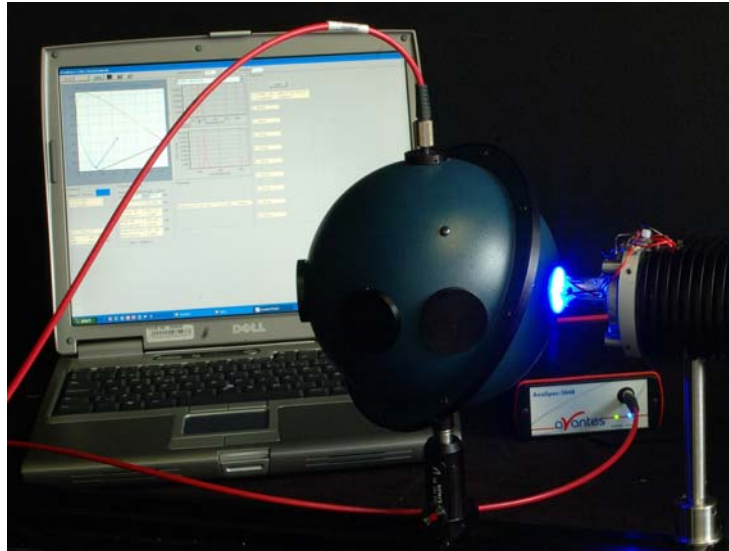
Figur 14 Spektrometrisk måleopstilling til måling af total udstråling fra enkelt high-power LEDs. En blå LED er monteret på en temperaturstabiliseret holder og alt lyset fra LEDen opsamles i en integrerende kugle.
