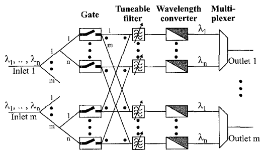
Fig. 2: OPEN OXC
