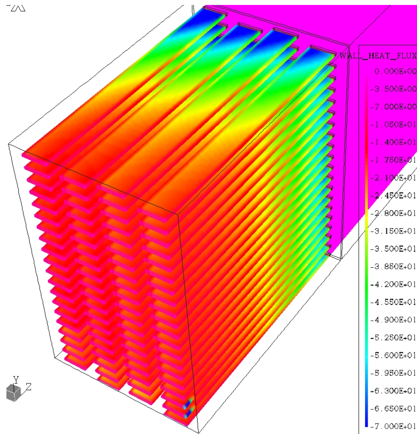
Figur 5.1.2c. Varmeflux [W/m 2 ] på finnerne i vekslersens varme del.
