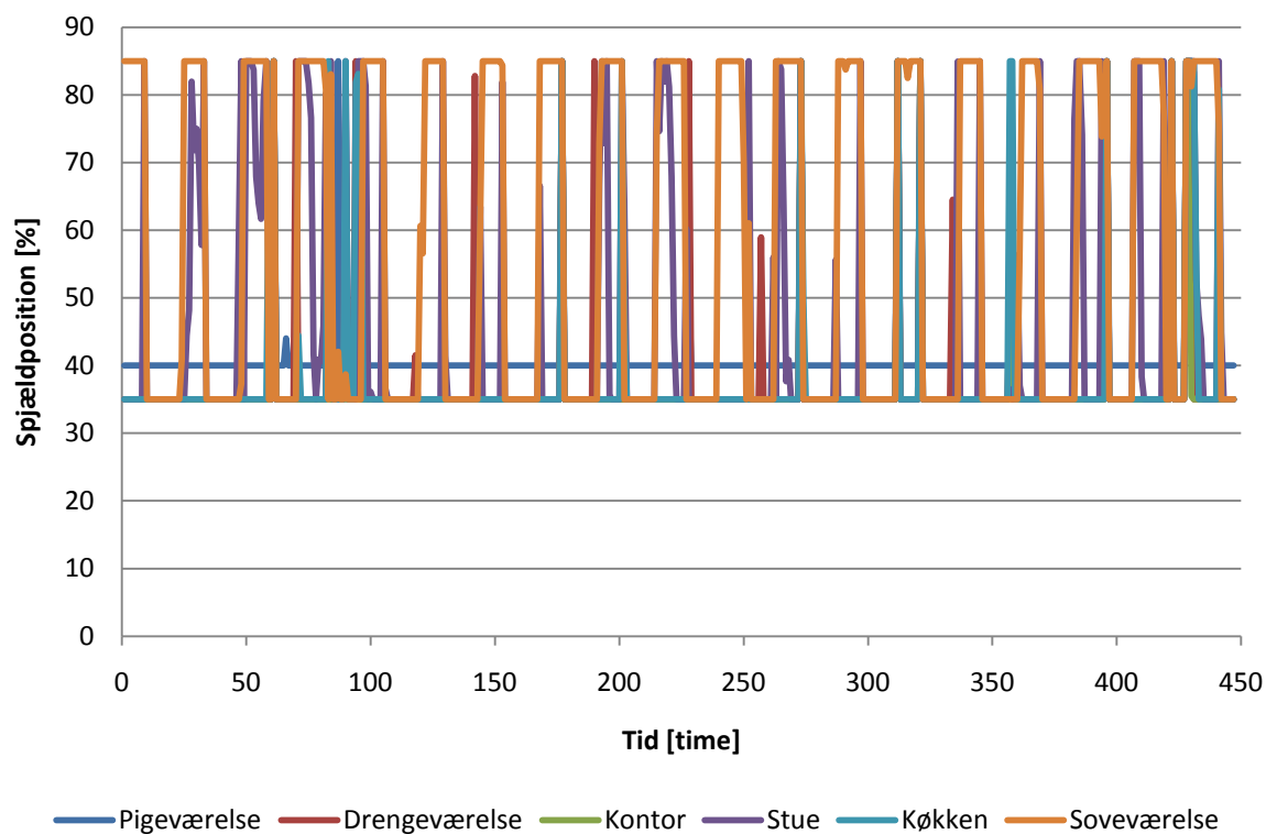
Figur 41. Spjældpositioner i måleperioden Avanceret 2 med CO 2 -setpunkt 800 ppm.
