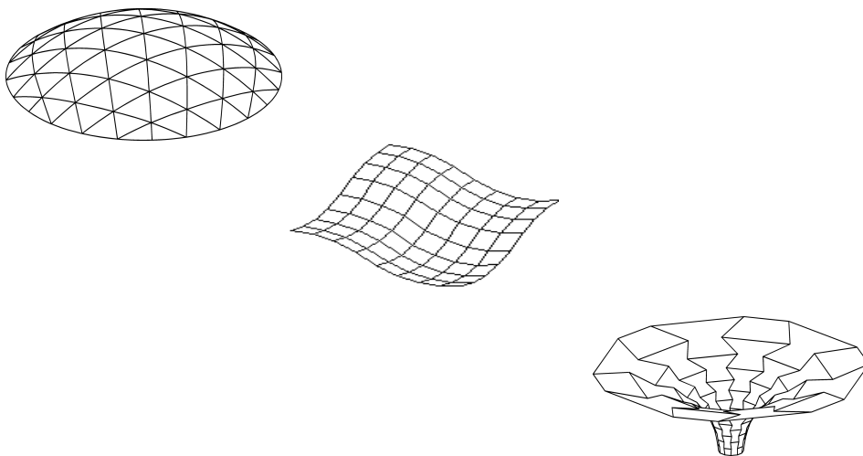
Figur 1. Eksempler på skaller opbygget af plane facetter: Gitterskal med trekantede facetter, hybrid- skal med firkantede facetter og firgrenede hjørner, samt skiveskal med tregrenede hjørner.
