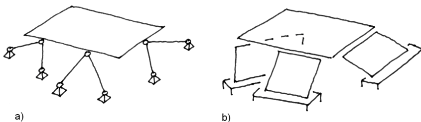
Figur 9. a) Et plant element er stabilt når det er fastholdt i tre punkter, således at det i hvert punkt er fastholdt i én retning, der ligger i elementets plan, og én retning, der skærer elementets plan. b) Et plant element er ligeledes stabilt hvis det er fastholdt af tre skiver, hvis planer alle skærer det betragtede elements plan og som hver er fastholdt som skive
