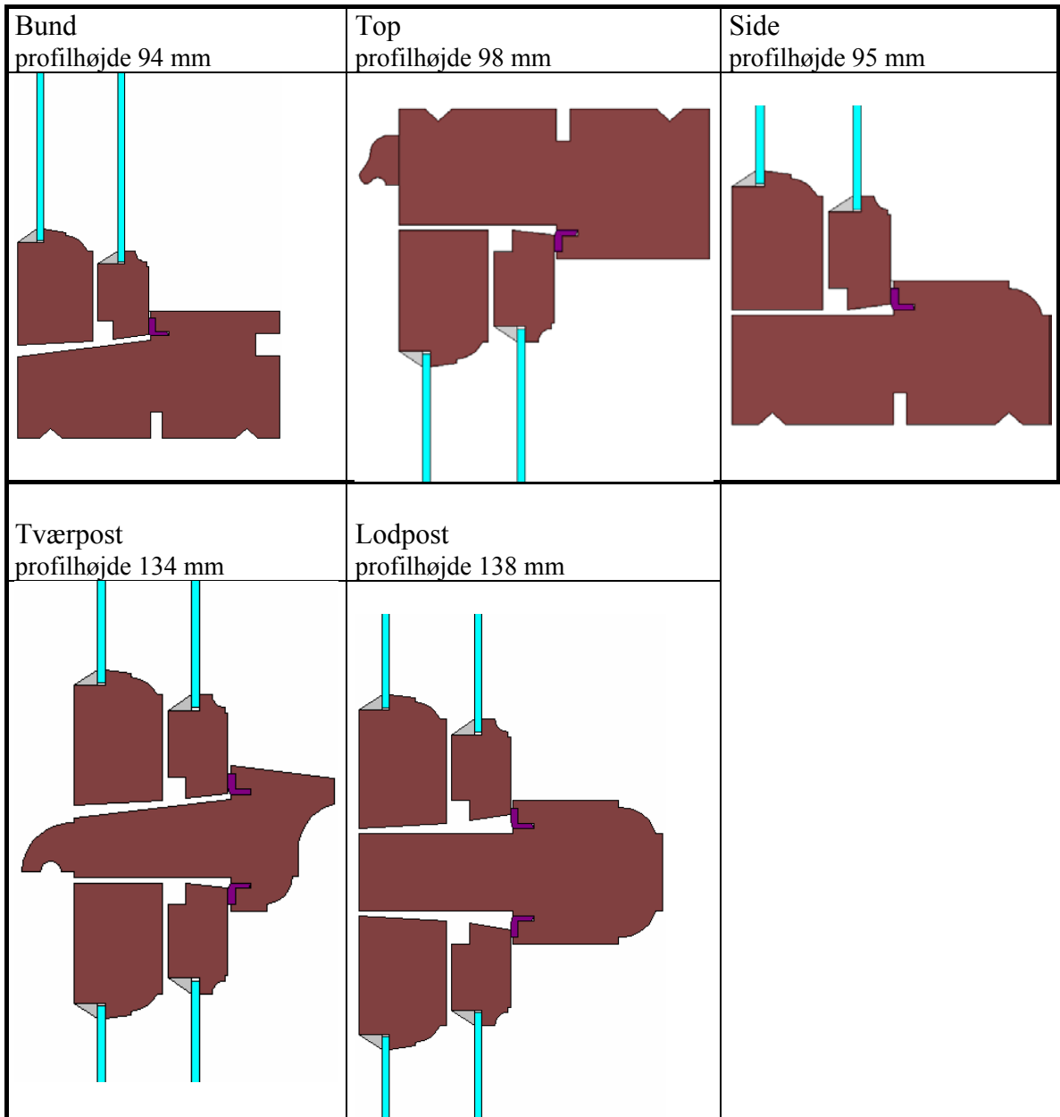
Figur 2. Profiler i vinduet med koblede rammer.
