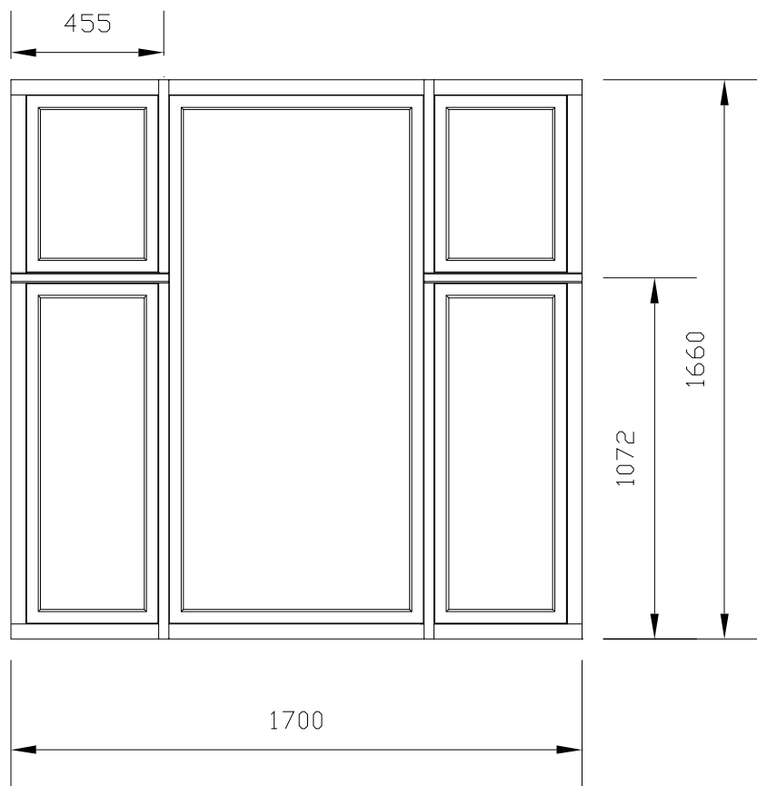
Figur 1. Udformning af de undersøgte frederiksbergvinduer. Mål i mm.
