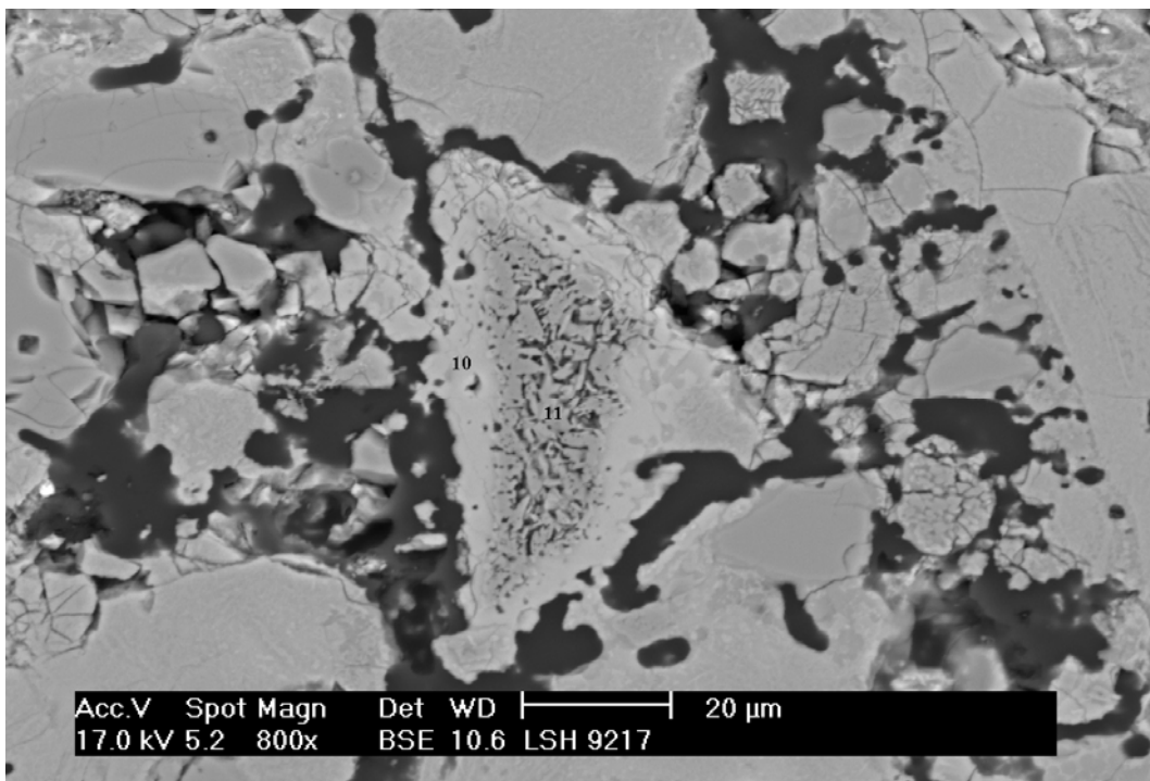
Figur 8. Fra prøven "Afbreakket klinke". Partikel i zone D. (11, Al_{39.8}Si_{0.2}O_{60} ) centralt af en porøs næsten ren aluminium oxid omgivet af en rand (10, Al_{15}Si_{15.8}Ca_{7.4}Na_{0.3}O_{61.5} ) af calcium aluminium silikat.
