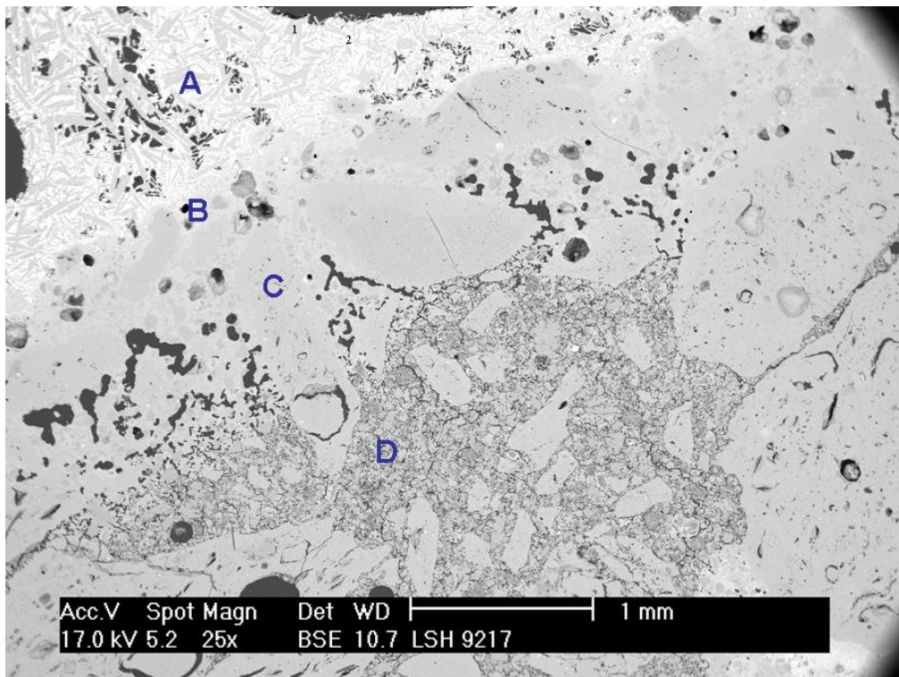
Figur 2. SEM billede af prøven: "Afbrækket klinke". Prøven er udtaget efter ca. 1300 timers forgasning i Viking. Der er markeret 4 karakteristiske zoner (se tekst) i materialet: Zone A: Indre varme zone, Zone B: Første overgangszone, Zone C: Anden overgangszone, Zone D: Centrale zone.
