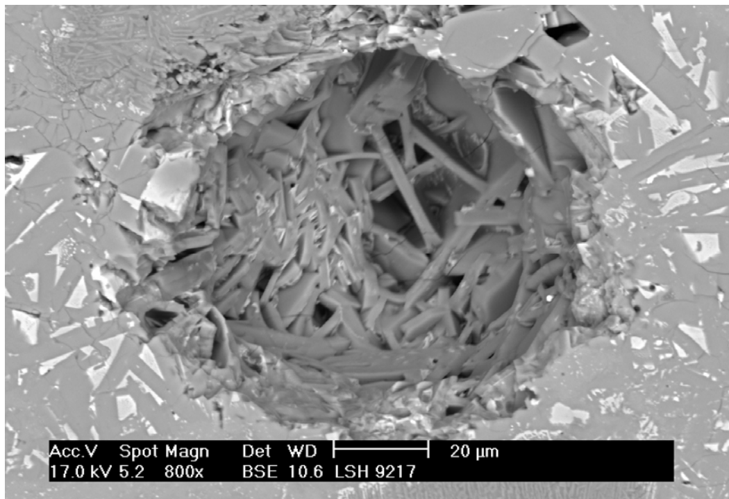
Figur 6. Nærbillede af dybereliggende pore fra afbrykket klinke i anden overgangszone, zone C. Den lamellerede skiftevis lyse og mørke zone er af typen, zone A.
