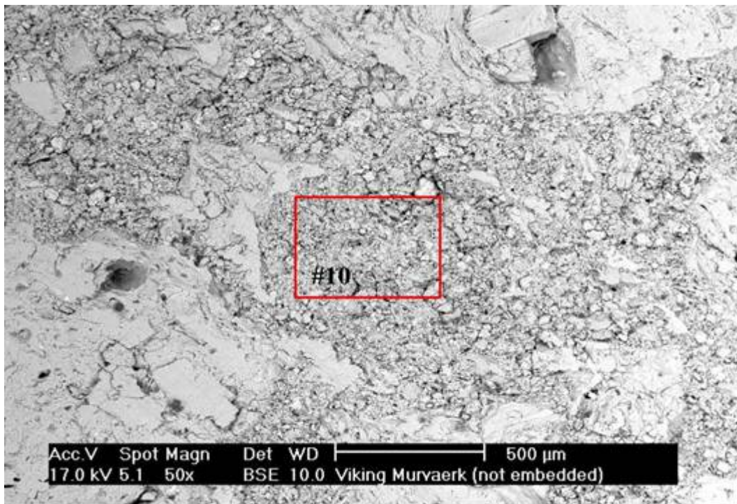
Figur 11. Centralt område fra prøven: "Murværkssten". [10, \text{Na}_{0.24}\text{Al}_{11.4}\text{Si}_{22}\text{Ca}_2\text{Ti}_{0.2}\text{Fe}_{0.3}\text{O}_{64}] Området er ikke indstøbt og af typen zone D.
