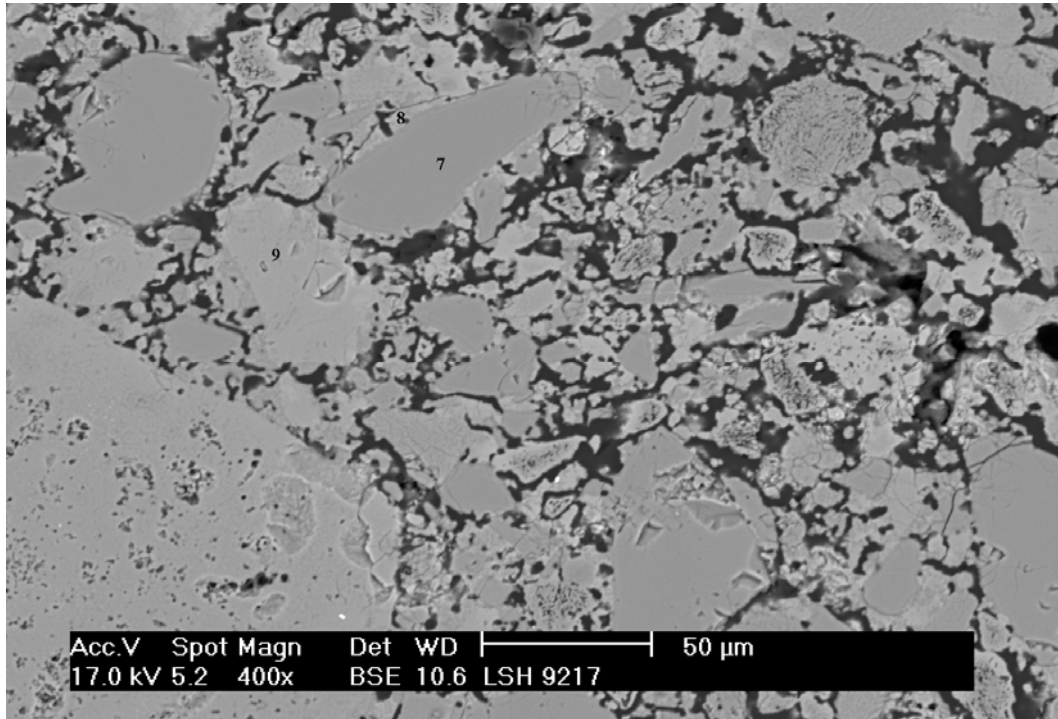
Figur 7. Fra prøven "Afbreakket klinke". Individuelle partikler i zone D. 7) Kvarts partikel 8) Kvartspartikel overflade beriget med natrium, calcium og aluminium, 9) aluminiumsilikat partikel.:
