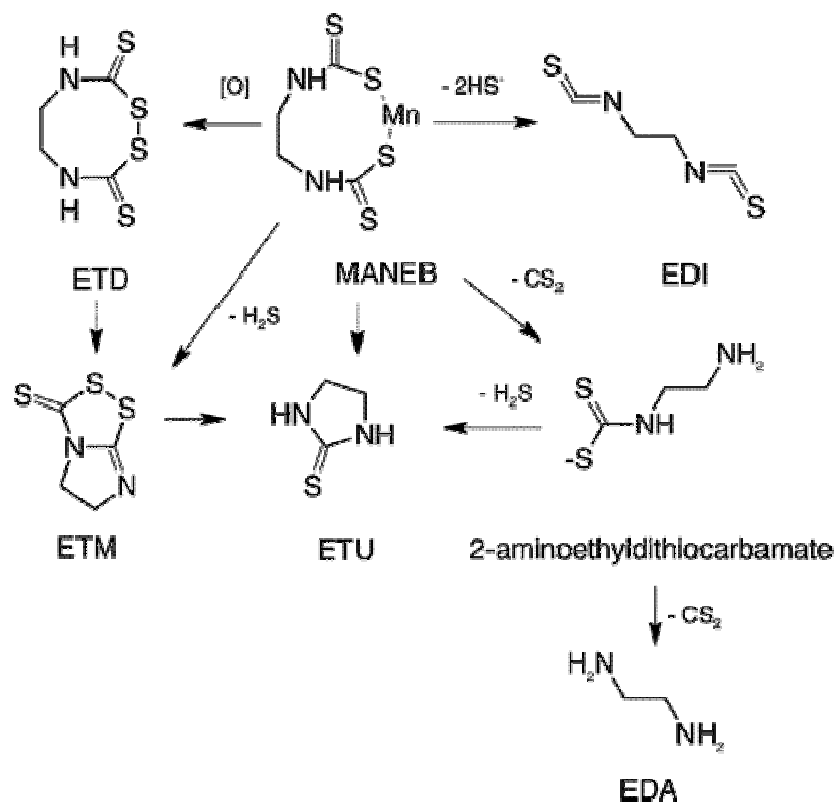
Figur 1. Foreslåede nedbrydningveje af maneb (som monomer) til ethylthiourinstof (ETU) og ethylendiamin (EDA) med følgende mulige intermediære nedbrydningsprodukter: ethylthiuram disulfid (ETD), ethylthiuram monosulfid (ETM), ethylendiisothiocyanat (EDI) samt 2-aminoethylthiocarbamat (Kontou et al. 2004)
