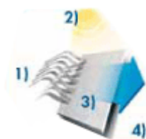
Fotokatalyse-principper
