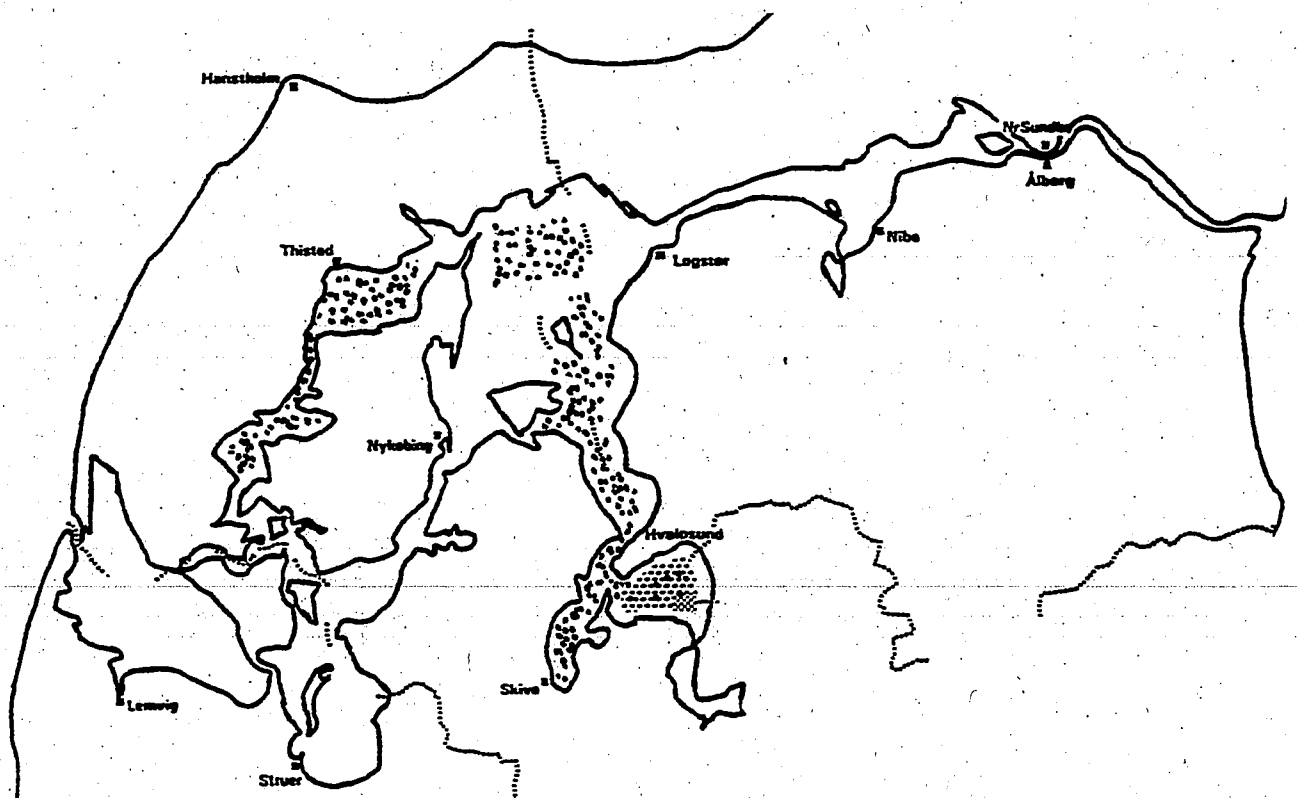
Figur 4. Udbredelsen af iltsvind sommerne 1994 og 1995. Kortene er udarbejdet af Limfjordsamterne.
