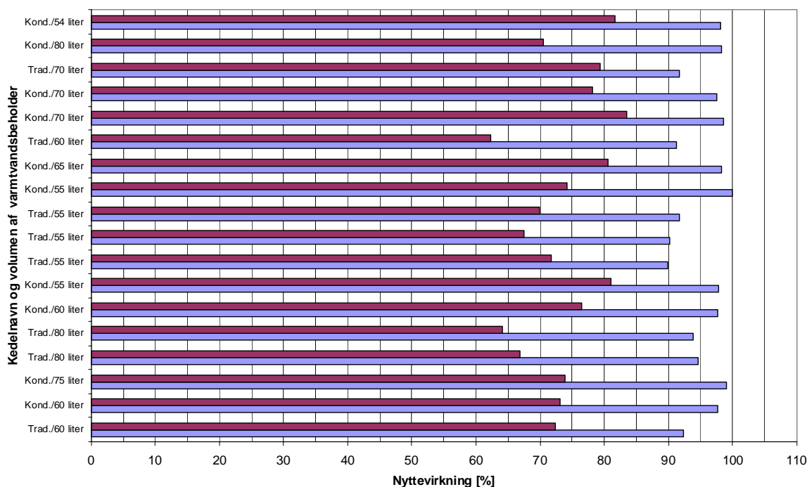
Figur 7. Nyttevirksomhed ved varmtvandsproduktion (3.000 kWh/år).
