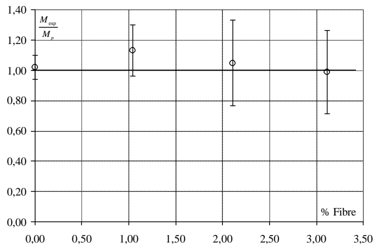
Figur 7.3 Resultater for ren bøjning med C25/30 beton
