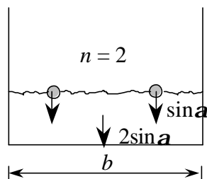
Figur 8.9 Brudmekanismen ved spaltebrud
