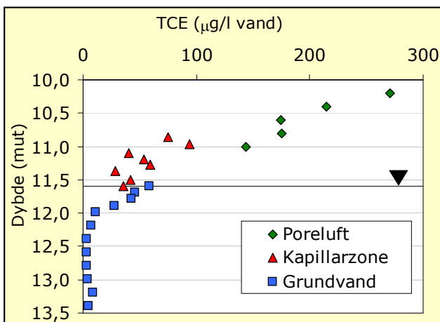
Observerede koncentrationer af TCE tæt på kildeområdet i poreluft, kapillarzonen og det øvre grundvand. Alle koncentrationer er omregnet til ækvivalente vand-koncentrationer.
