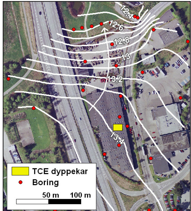
Potentialekort i det sekundære magasin for området omkring Rundforbivej 176. Pejledata er fra marts 2006. Strømningsretningen er nordøstlig.
