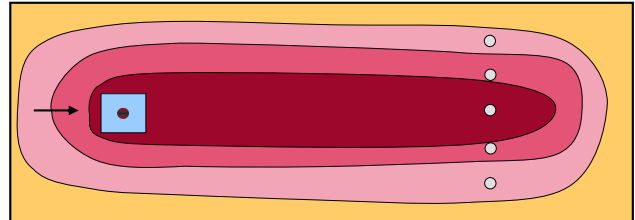
Figuren illustrerer den konceptuelle model for forureningsspredningen ved Rundforbivej 176 i et langsgående snit og en plantegning. Spildet af TCE forårsager spredning med to mekanismer. Gasspredningen giver en bred forureningsfane, mens den formodede spredning som fri fase giver en smal og dyb forureningsfane.
