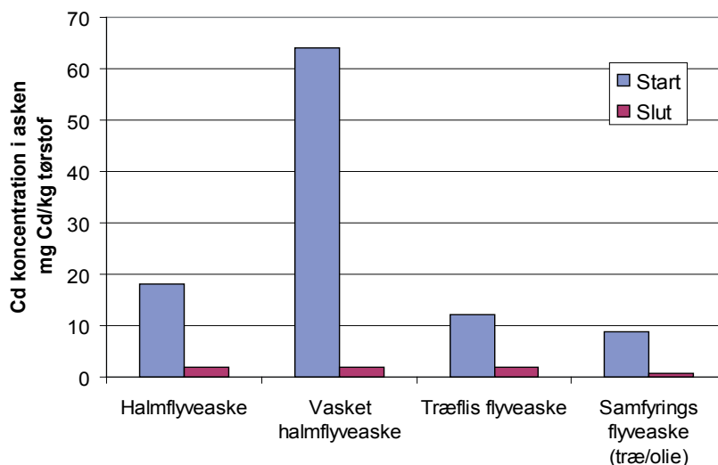
Ovenstående figur viser cadmium-koncentrationen i forskellige bioaske før og efter elektrodialytisk rensning. Resultater fra laboratorie-skala forsøg.
