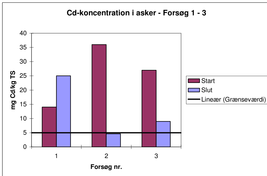
Figur 7: Start- og slutkoncentrationer af cadmium i asker samt grænseværdi – rensningsforsøg nr. 1 – 3.
