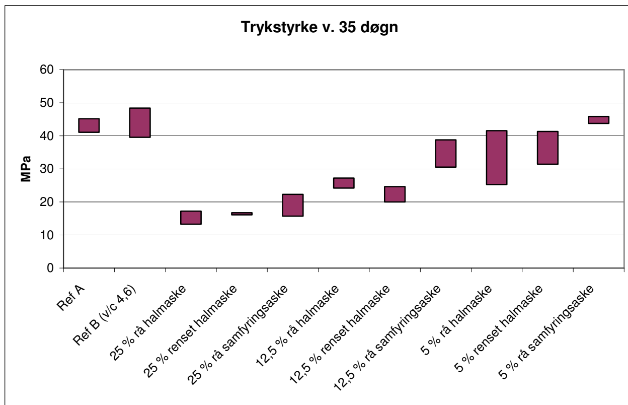
Figur 13. Trykstyrke af mørtelprøver, megapascal (MPa) efter 35 døgn hærdning (dog 34 dage for 12,5 % rå halmáske). Resultaterne er afbildet som et interval omkring middelværdien af 3 prøveemner (6 for reference A) +/- standardafvigelsen.
