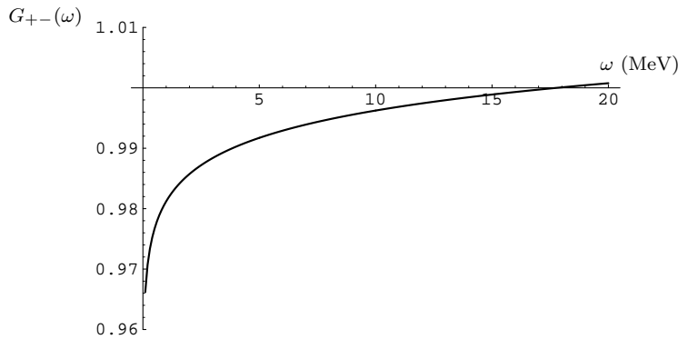
FIG. 2. The function G_{+-}(\omega) .
