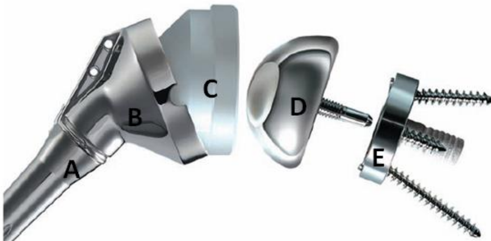
Fig 19. Components de la pròtesi invertida d'espatlla: (A) diàfisi, (B) epífisi, (C) polietilè (D) glenosfera, (E) metaglena 38 .
