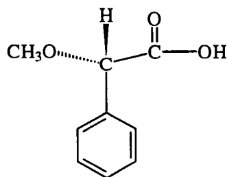
Figura 11-10: Àcid ( S )-(+)- \alpha -metoxifenilacètic (MPPA): (51)
