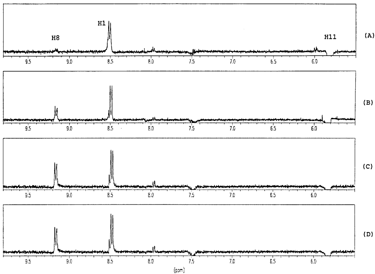
Espectre 7-27: Espectres NOE del 9-antril- iso -propilcarbinol (4) a diferents temperatures després d'irradiar el protó H 11 durant 8 segons a la potència de 50 L; (A), espectre a 210 K, (B), espectre a 225 K, (C), espectre a 235 K i (D), espectre a 245 K
