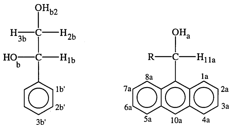
1-fenil-1,2-etandiol
