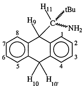
Figura 11-15 : 9-(1-amino-2,2-dimetilpropil)-9,10-dihidroantracè: (53)
