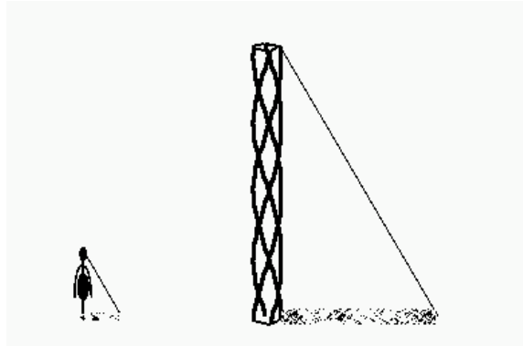
Figura 2: Semblança de triangles
