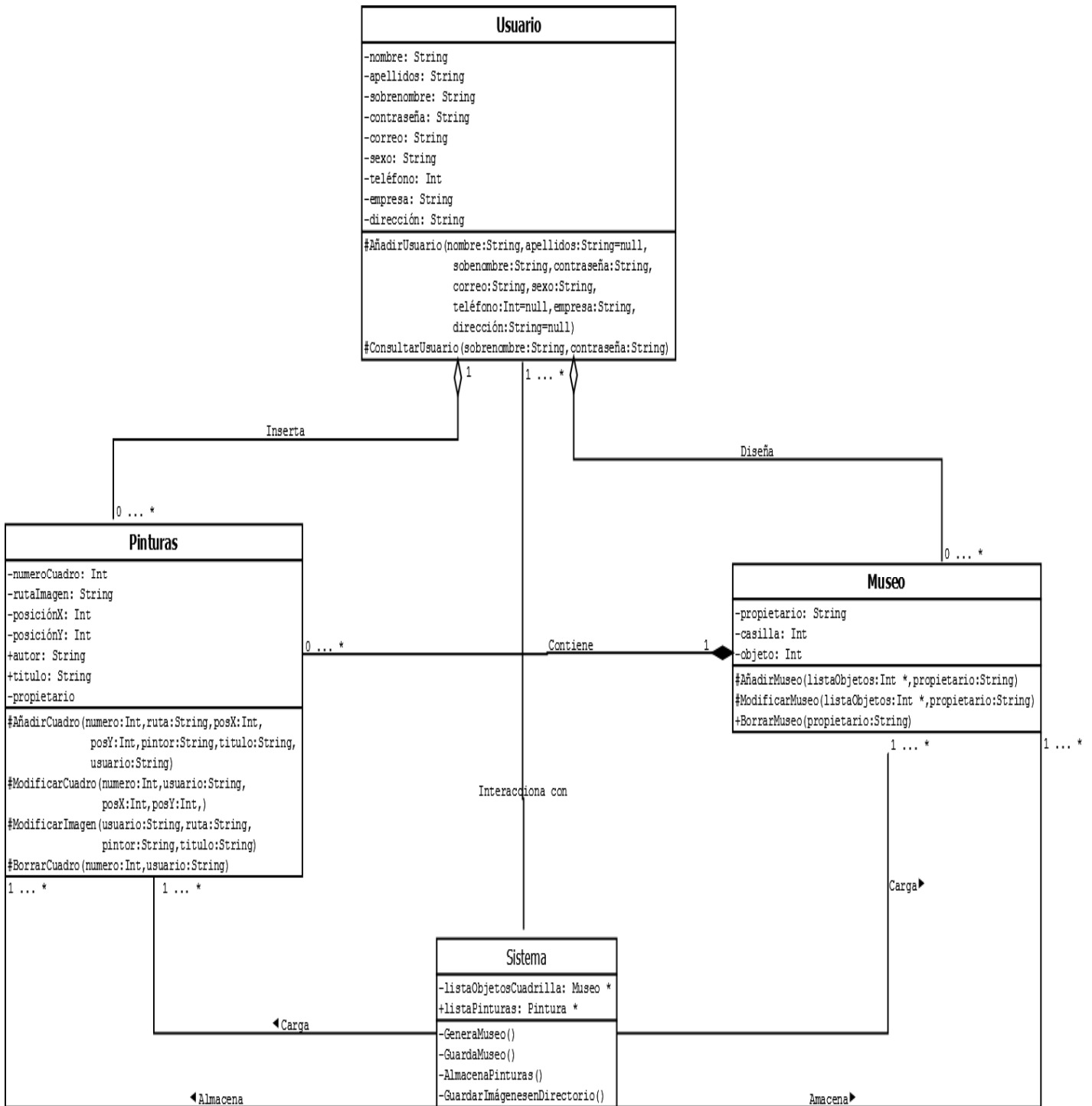
Figura 6. Diagrama de las clases “Generador de museos virtuales en navegadores web”
