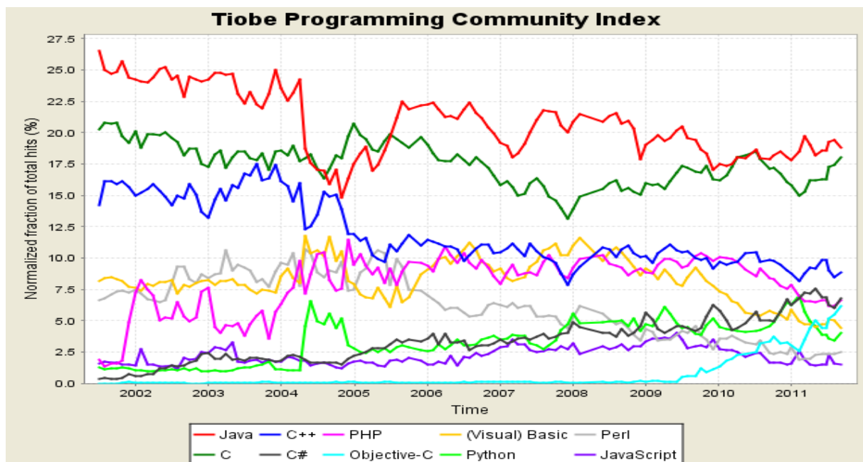
Figura 1. Tendencias a largo plazo en el Top 10 de los lenguajes de programación.
