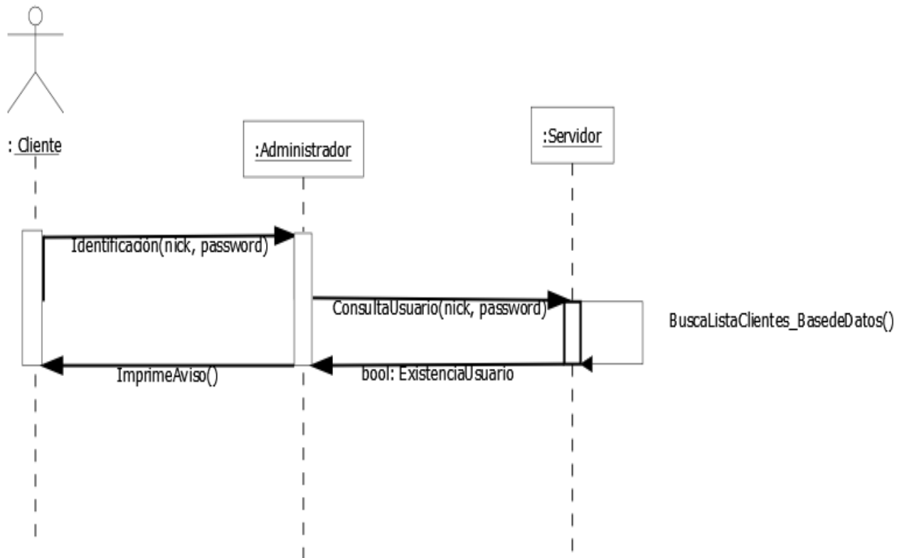
Figura 5. Diagrama de secuencia “Iniciar Sesión”.
