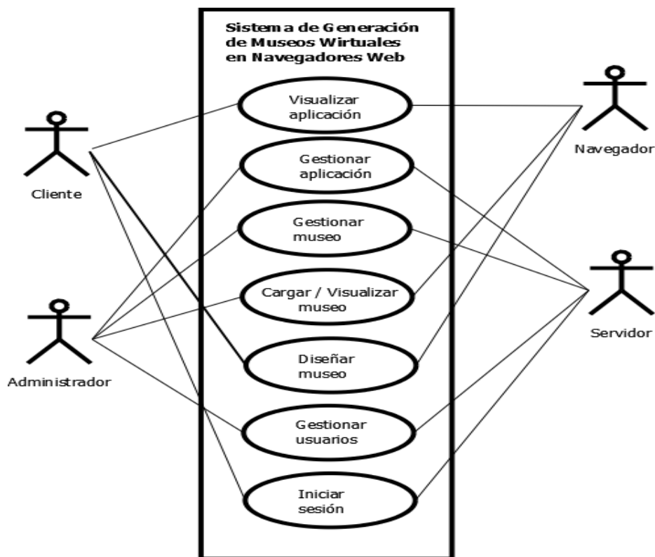
Figura 3. Diagrama Caso de Uso “Generación de Museos Virtuales para Navegadores”
