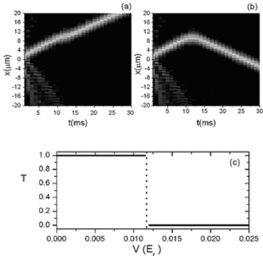
Fig.1- Mapa de contorn de l'evolució en espai i temps d'un solitó de gap interaccionant amb una barrera de potencial efectiva en condicions per a les que es produeix (a) efecte túnel o (b) reflexió. (c) Coeficient de transmissió, T, en funció de l'alçada de la barrera de potencial efectiva.
