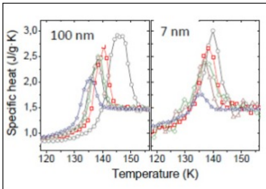
Calor específica en funció de la temperatura per capes primes de toluè per alguns temps d'envelliment seleccionats a una temperatura de 90 K. Equerra: 100nm de gruix, dreta: 7nm de gruix. Estrella blava: capa refredada ràpidament a partir del líquid; triangle marró: temps d'envelliment (a 90K) de 5 min; rombe verd: 30 min; quadrat vermell: 720 min; cercle negre: dipositat a partir de fase vapor (color online).
