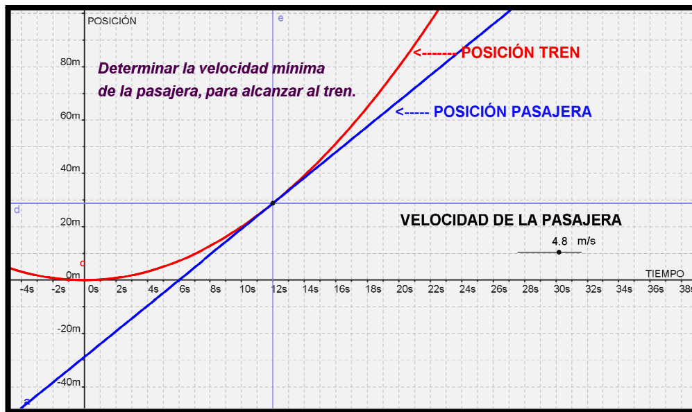
Figura 1: Solución del problema de cinemática utilizando el GeoGebra.
