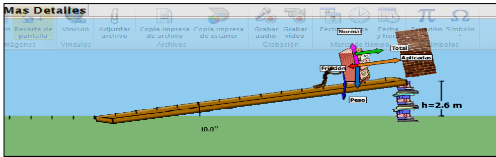
Figura 2: Pantalla del software PhET, sobre dinámica del movimiento en un plano inclinado.
