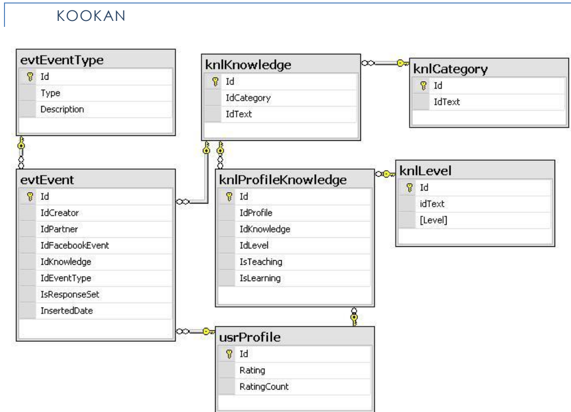
Figura 9 – Base de dades de Kookan
