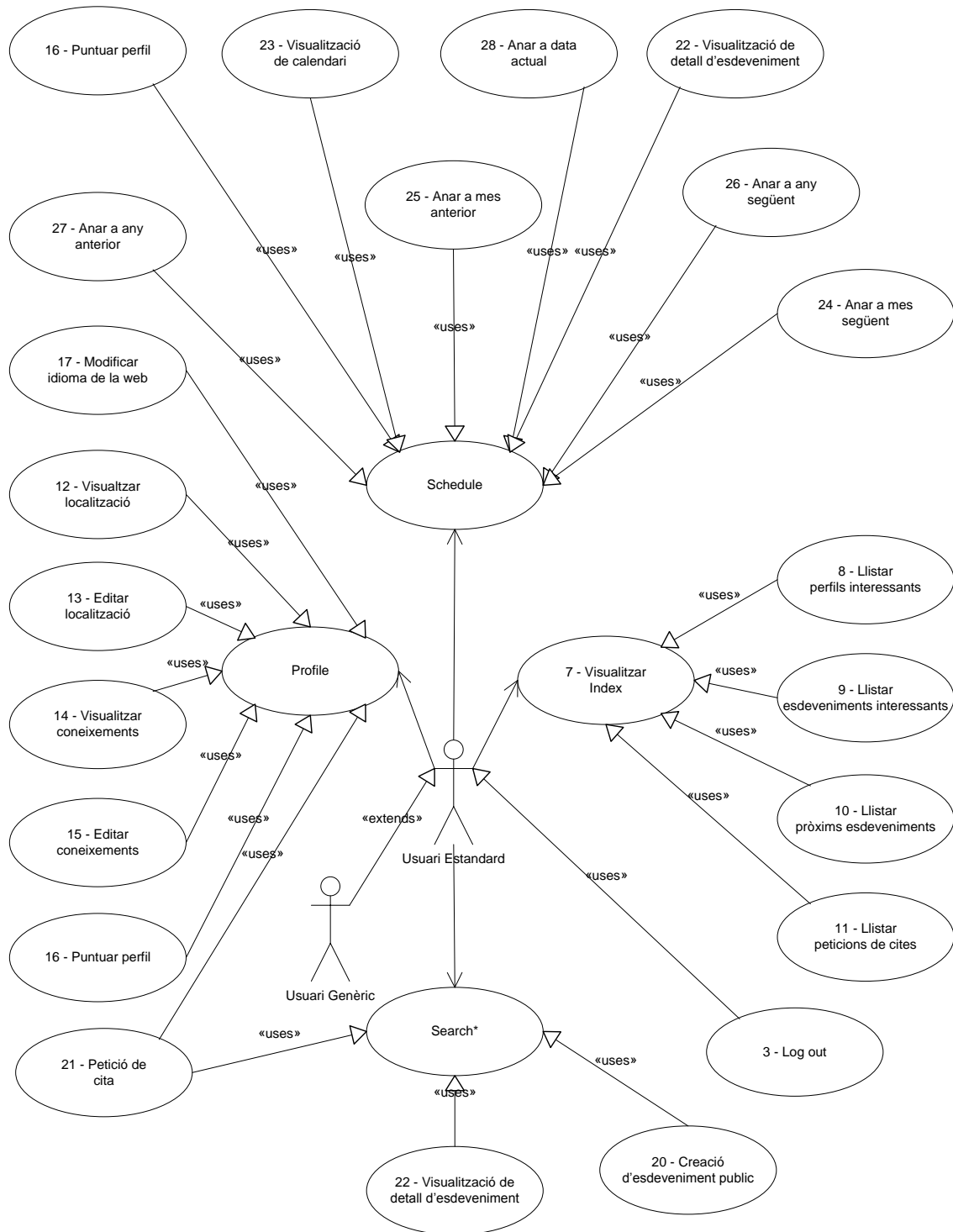
Figura 5 – Casos d'ús de l'usuari estàndard
