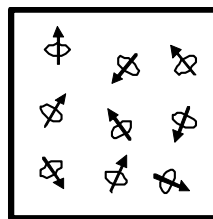
a. Material paramagnètic en absència de camp magnètic.
