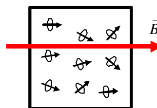
b. Material paramagnètic sota l'acció d'un camp magnètic aplicat.
