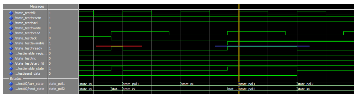
Figura 6.2: Waveform de la unidad de control durante la recepción.
