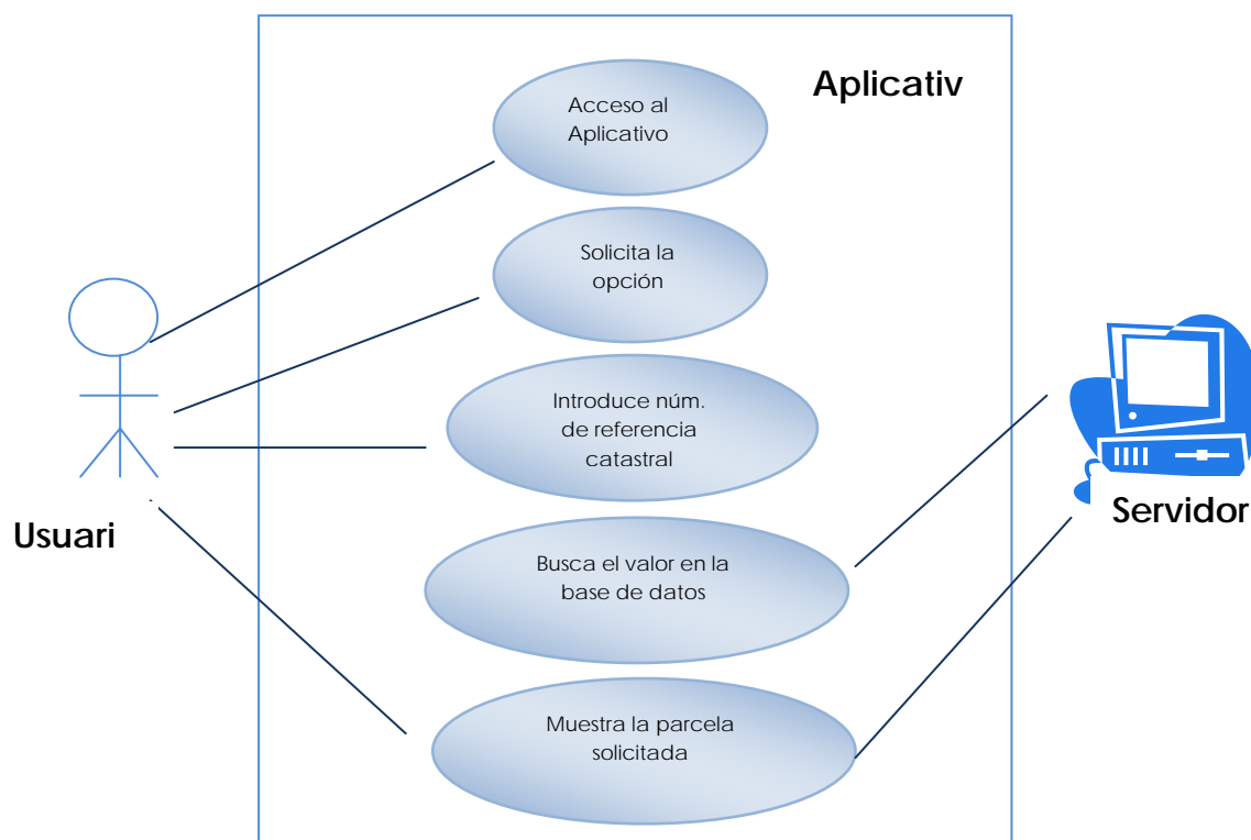
Figura 8. Caso de uso de localización de parcela por referencia catastral
