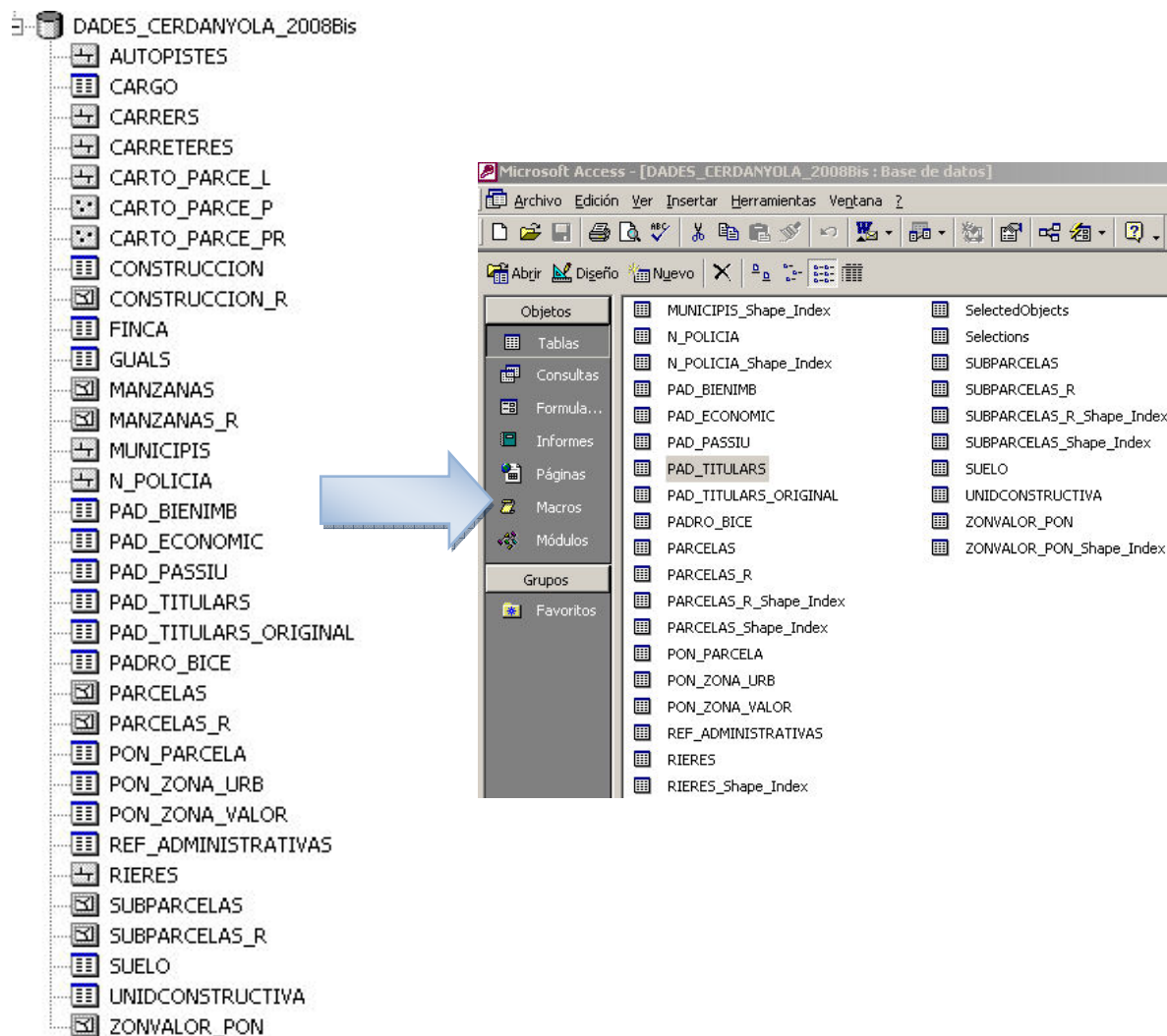
Figura 5. Estructura de la Geodatabase personal local existente
