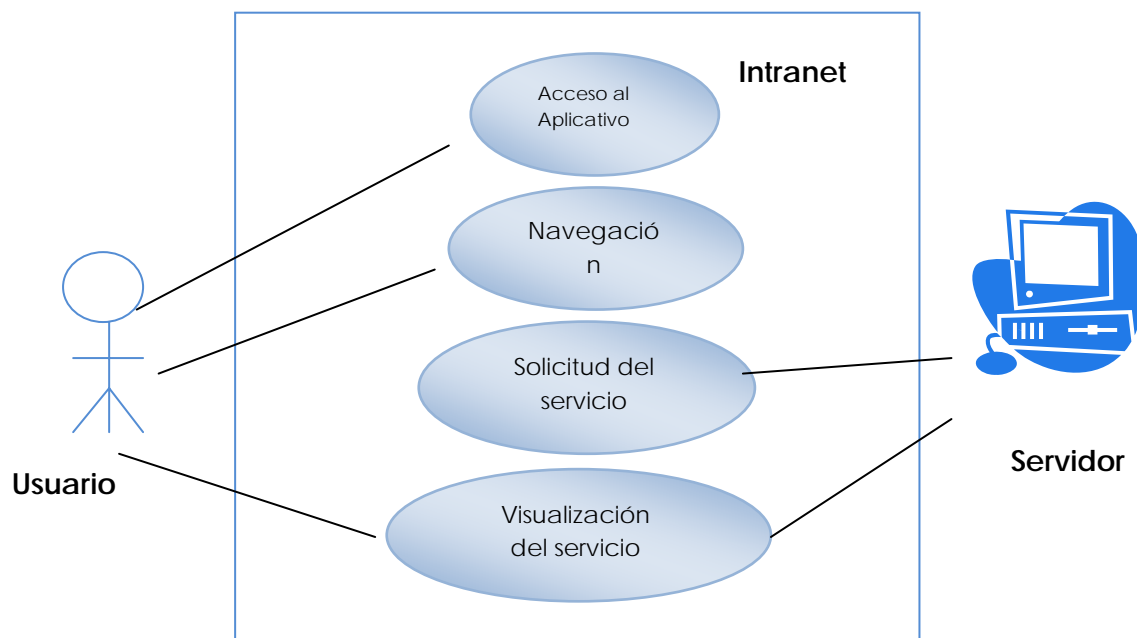
Figura 7. Caso de uso de la visualización del Aplicativo web Intranet
