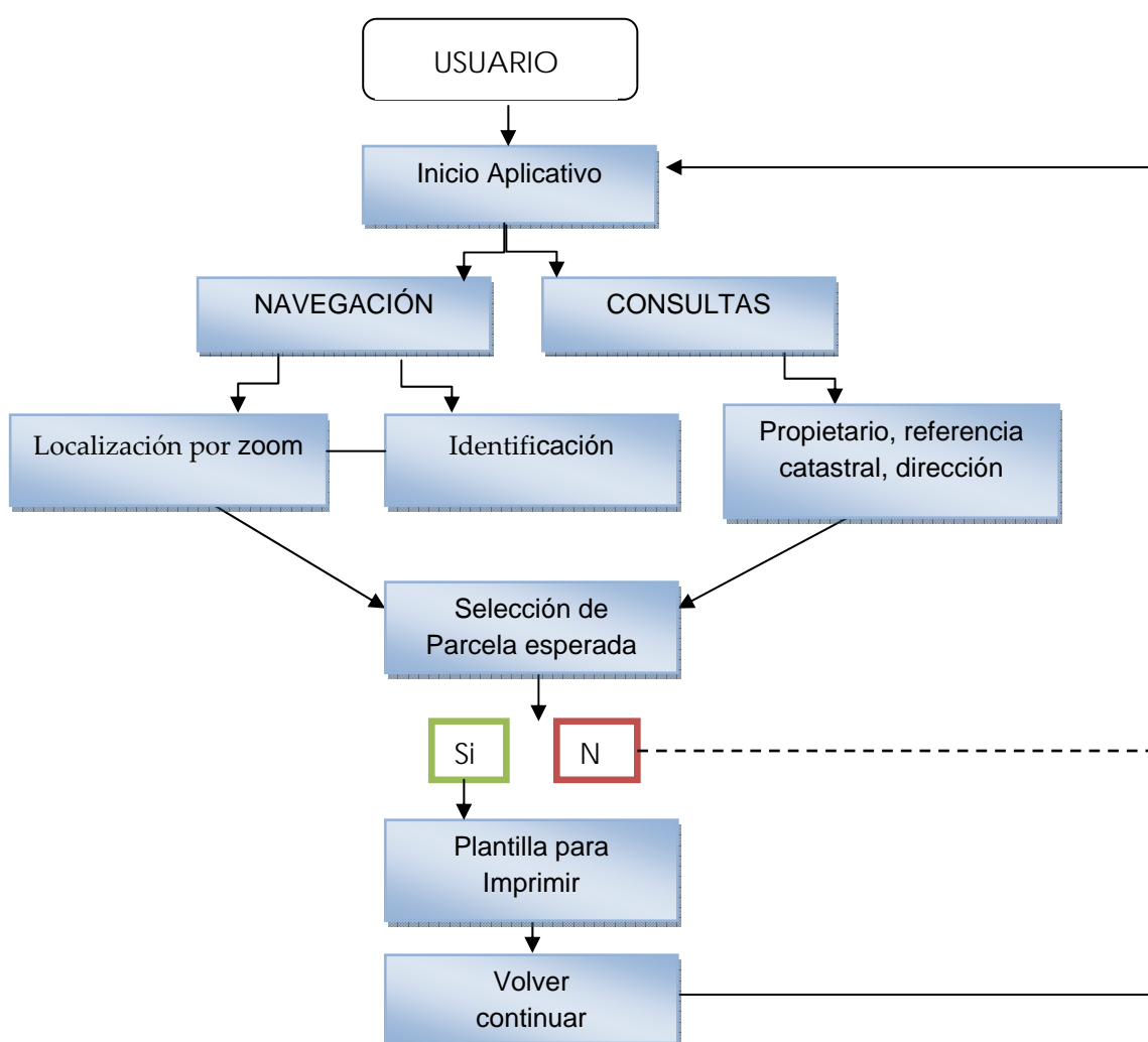
Figura 15. Diagrama que representa la utilización de la aplicación
