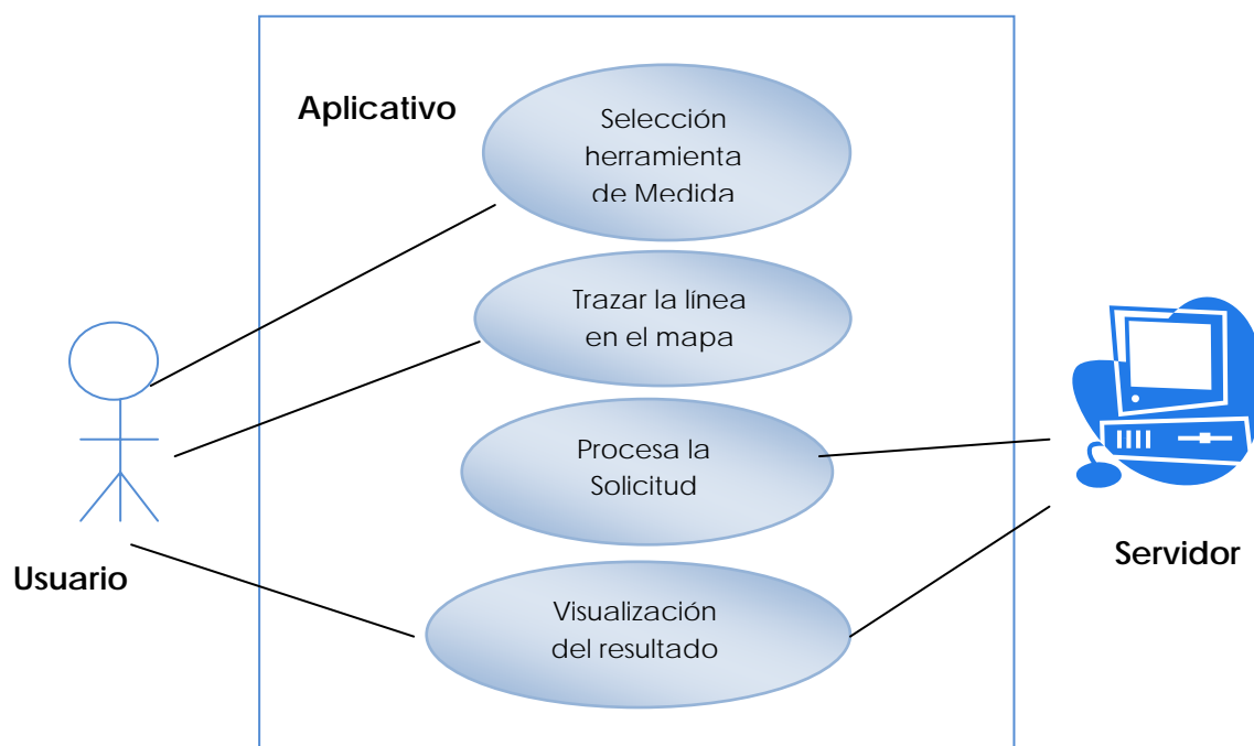
Figura 9. Diagrama de caso de uso de la herramienta de medir distancia en el mapa
