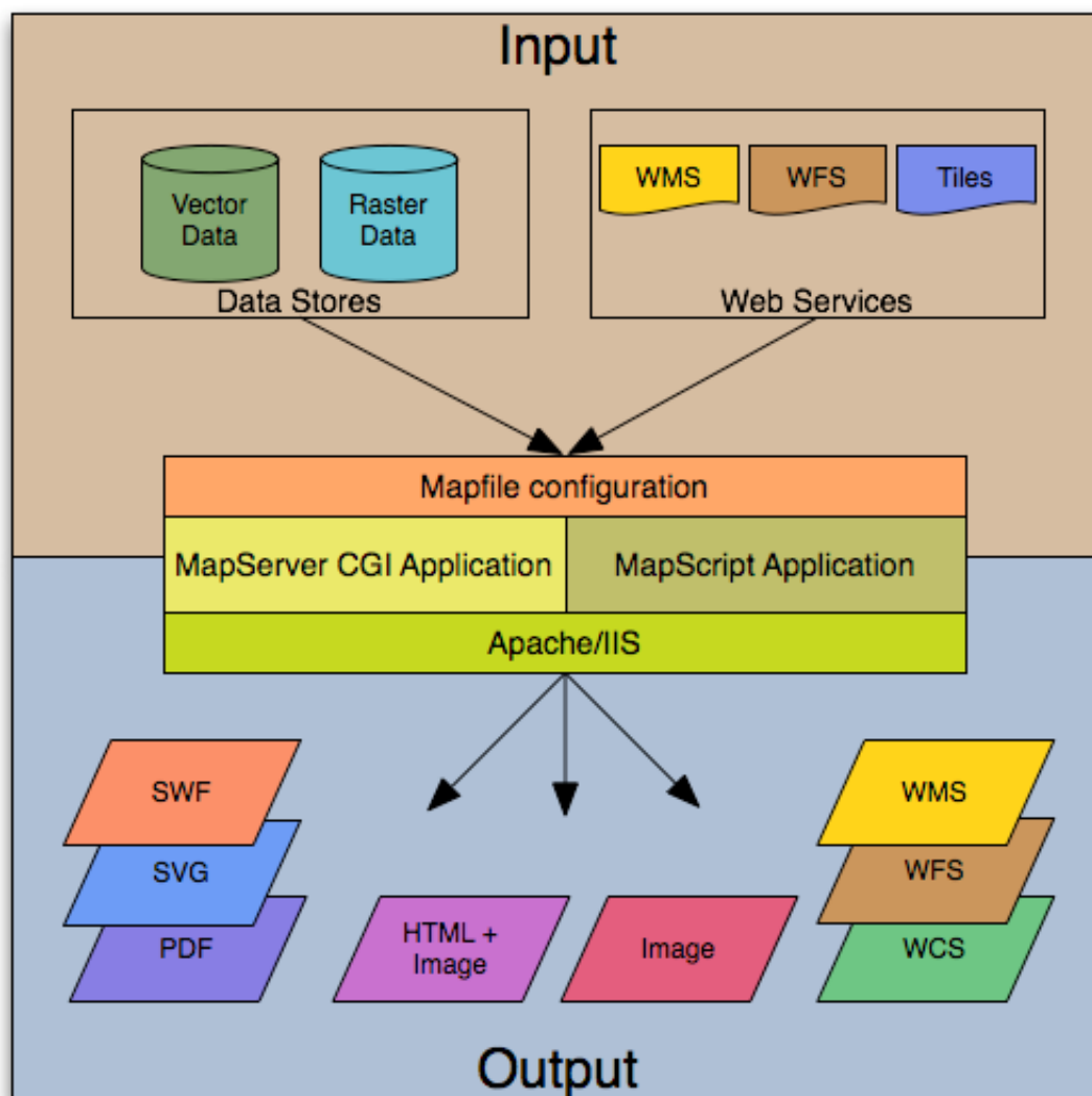
Figura 6. Arquitectura básica de una Aplicación MapServer
