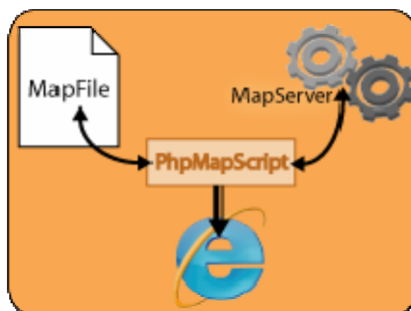
Figura 16. Funcionamiento PHP con MapServer
