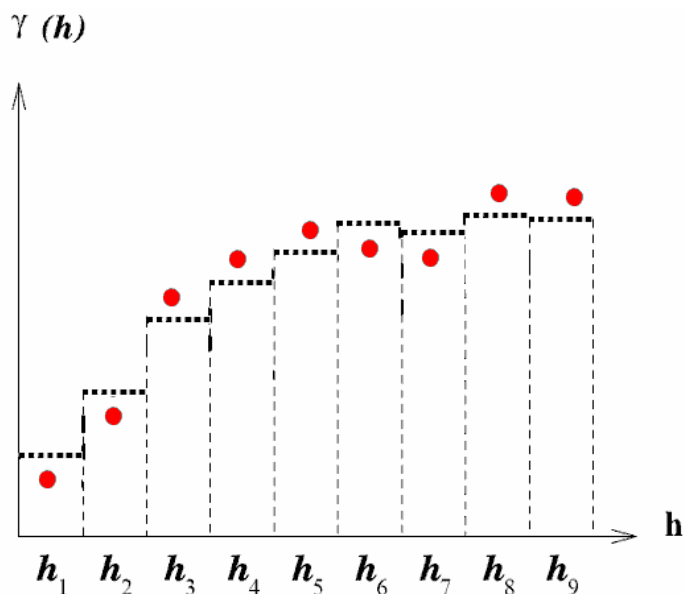
Figura 2.3: Segon pas de la generació del variograma empíric: càlcul i representació de la diferències quadràtiques promitjades agrupades per intervals de separacions h
