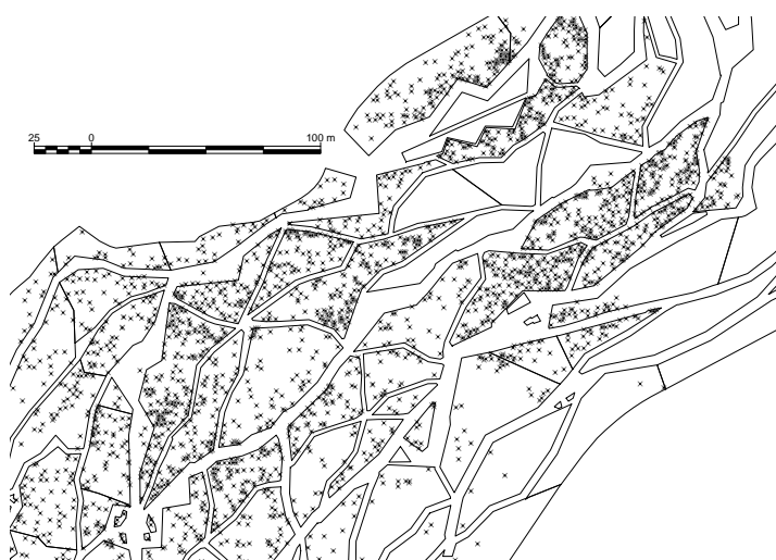
Figura 5.8: Vista parcial de la distribució de la mostra amb valors altitudinals.
