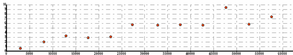
Figura 3.2: Variograma empíric amb 12 intervals d'amplada 5000 m.
