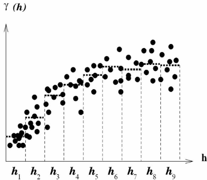
Figura 2.2: Primer pas de la generació del variograma empíric: càlcul i representació de la diferències quadràtiques de parells de dades en funció de la seva separació h .
