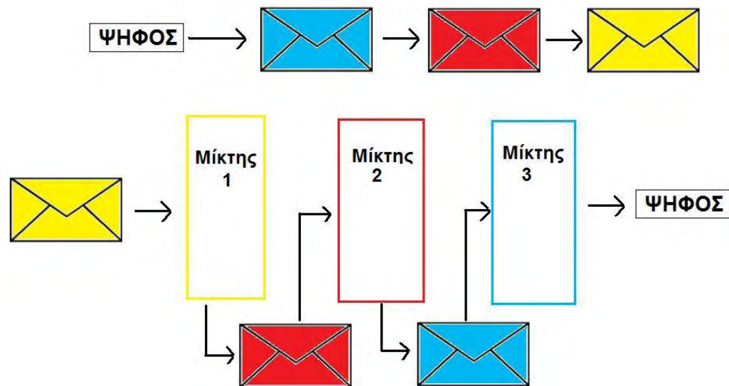
Εικόνα 3. Παράδειγμα Mix-net αποκρυπτογράφηση
