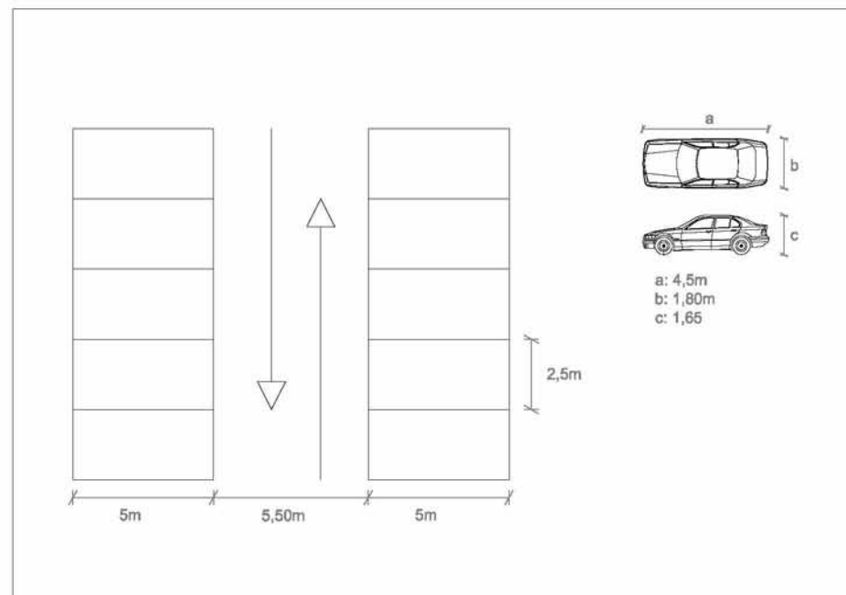
Απαιτούμενες διαστάσεις χώρου στάθμευσης
