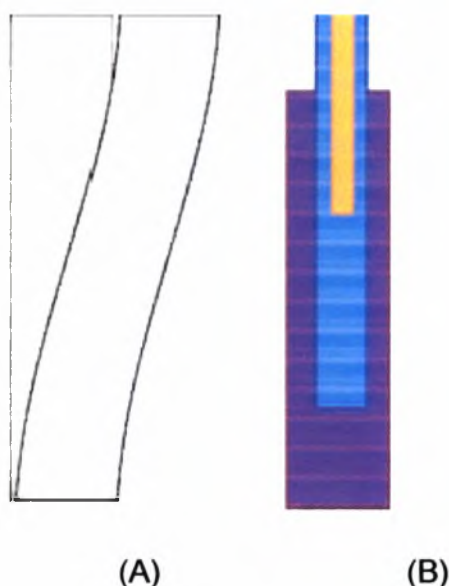
Σχήμα 2.17 Σχηματική απεικόνιση των δύο πιθανών τρόπων παραμόρφωσης και αστοχίας των νανοσωλήνων. (Α) Λυγισμός σε μια λεπτή στήλη. (Β) Τηλεσκοπική ενός Πολύτοιχου νανοσωλήνα. Η θραύση των νανοσωλήνων είναι ο τρίτος τρόπος, αλλά δεν εμφανίζεται στο σχήμα.
