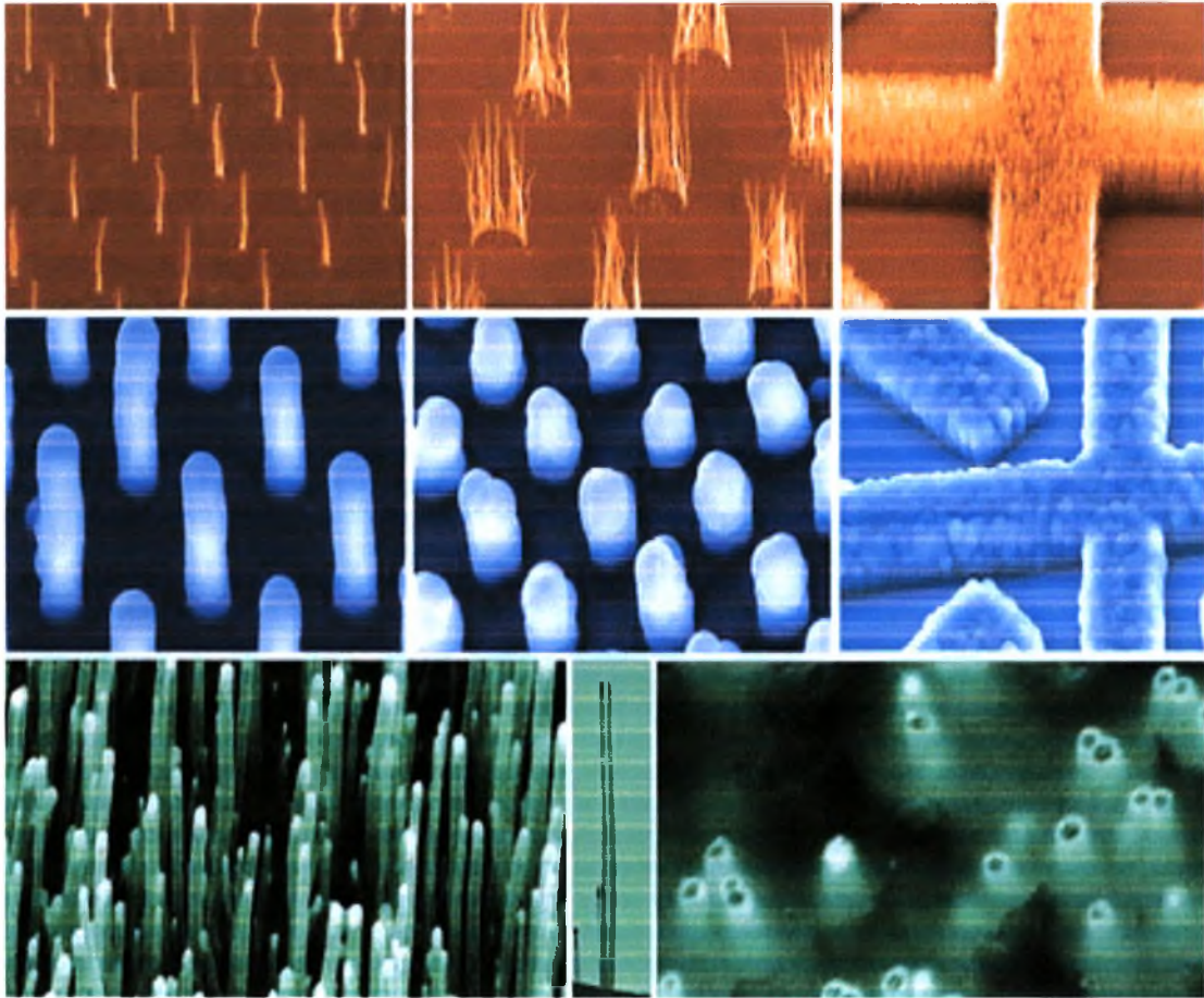
Σχήμα 2.14 Νανοσωλήνες (NASA, 2008)
