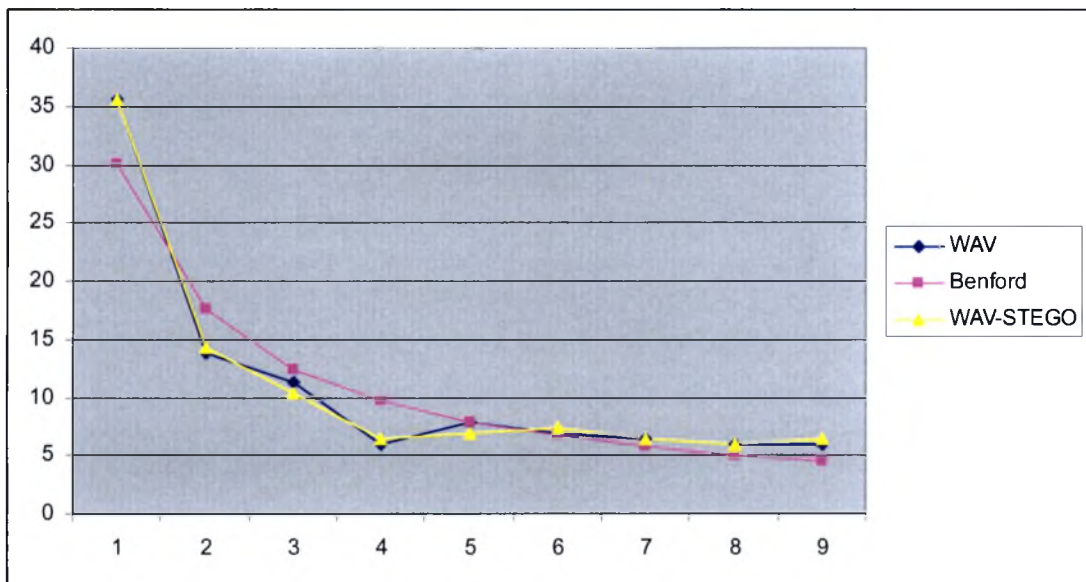
Εικόνα 5.2: Αρχείο WAV
