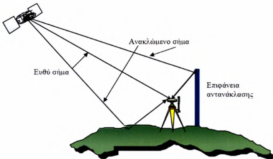
Σχ.6.3. Το φαινόμενο τις πολυδιαδρομής (multipath)
