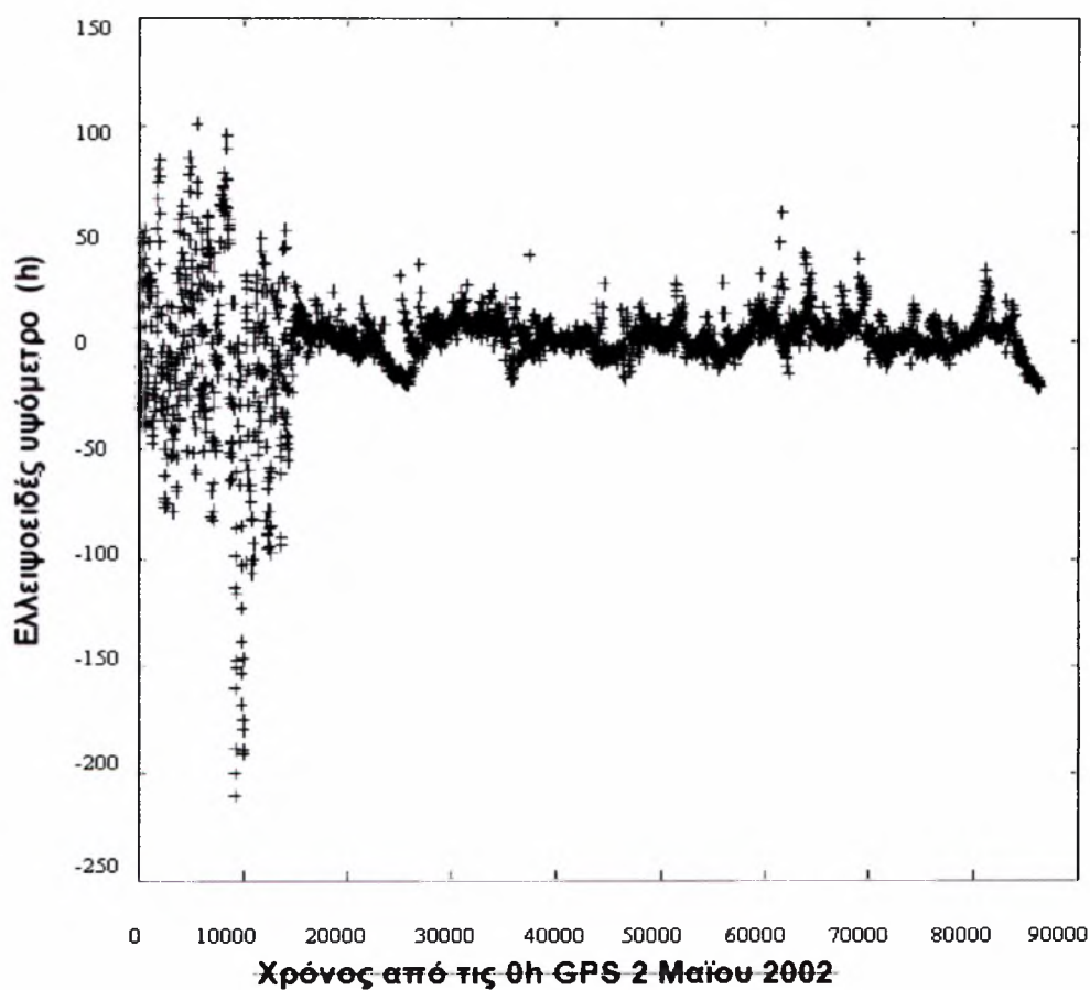
Σχ. 3.3. Παράδειγμα προσδιορισμού υψόμετρου (h) σημείου με GPS, με SA αριστερά χωρίς SA δεξιά
