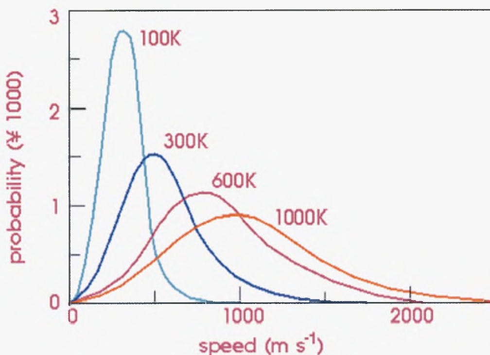
Εικόνα 11. Η κατανομή Maxwell για την ταχύτητα των ατόμων ενός συστήματος σε διάφορες θερμοκρασίες [15].
