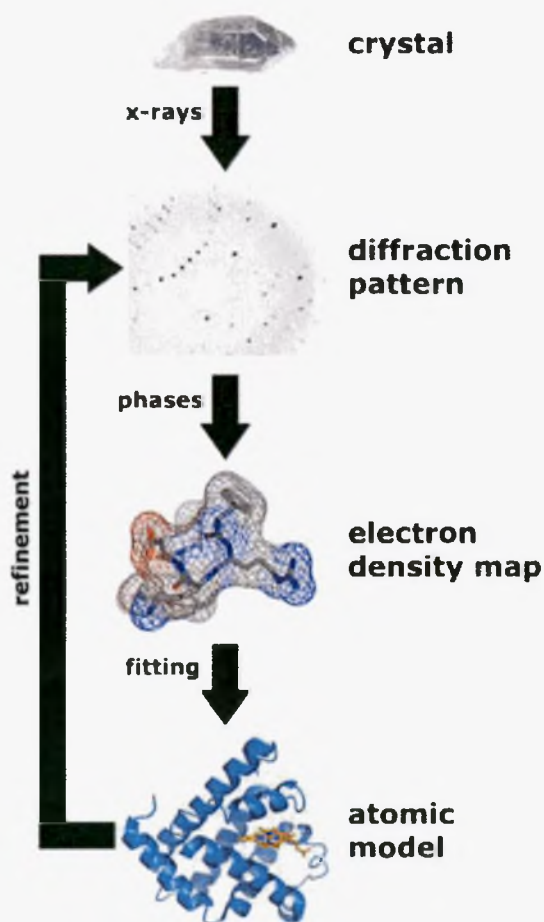
Εικόνα 4. Απλοποιημένο διάγραμμα της διαδικασίας που ακολουθείται για τον προσδιορισμό της δομής μιας πρωτεΐνης, με την μέθοδο της κρυσταλλογραφίας με ακτίνες X [7].
