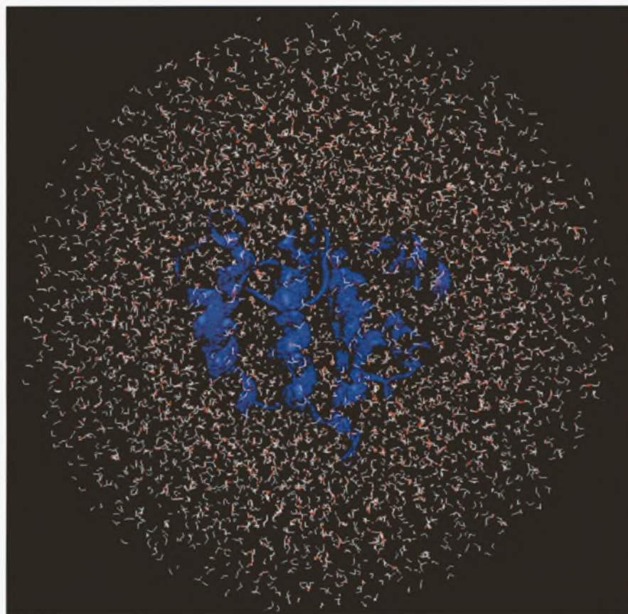
Εικόνα 12. Η πρωτεΐνη RanGAP1 περιβαλλόμενη από μία σφαίρα νερού.
