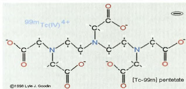
Εικόνα 1: 99m Tc
