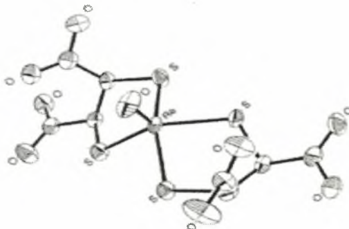
Εικόνα 5: ^{188}\text{Re-DMSA}
