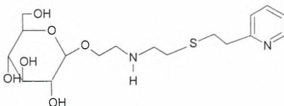
Εικόνα 11: 2-N-ethyl-β-D-glucopyranose-2-[(2-pyridine-2-ylethyl)thio]ethanamine
