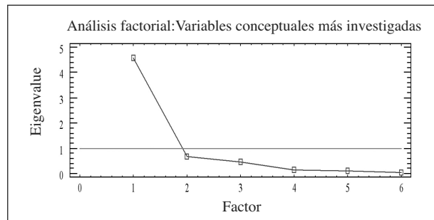
Figura 2 Análisis factorial de las variables conceptuales más indagadas.
