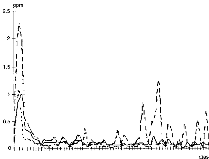
Figura 1. Evolución de la concentración de amonio total respecto al tiempo para cada uno de los tanques. Tanque control, línea continua; Alken Clear Flo 1200, línea discontinua, y Biozyme, línea punteada.
