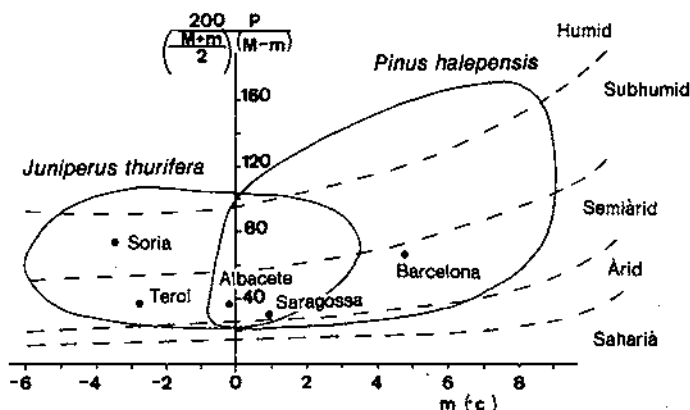
Figura 7. Localitats de Juniperus thurifera i de Pinus halepensis en el climatograma d'Emberger, segons Quézel (1976) i Sébastian (1965), lleugerament modificat. L'abscissa ( m ) és la mitjana de les mínimes del mes més fred. L'ordenada és el quocient pluriotèrmic d'Emberger, on P és la precipitació anual (en mm) i M és la mitjana de les màximes del mes més càlid. Observi's l'aridesa extrema de Saragossa.
