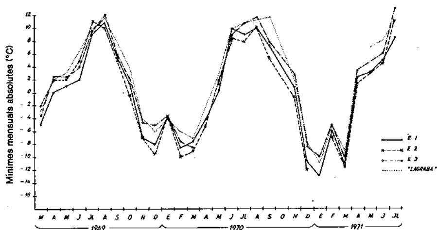
Figura 4. Mínims mensuals absoluts de la temperatura de l'aire a la Retuerta de Pina. Les estacions E1 i E2, al fons d'una val, tenen generalment mínims inferiors a les de E3 i Lagraba (20-50 m pel damunt de les primeres).
