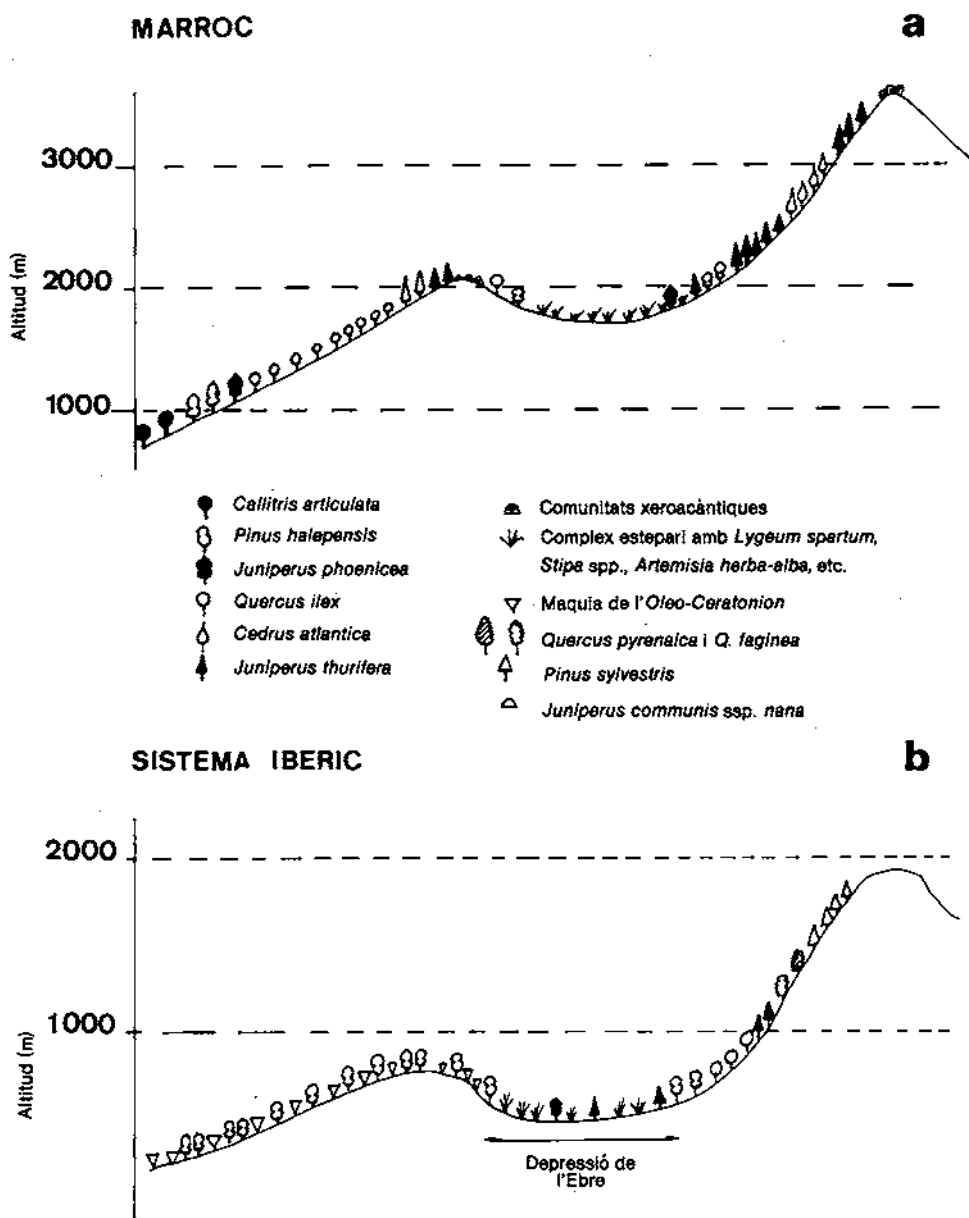
Figura 8. Sèries altitudinals comparades. (a) Transecte nord-sud del Gran Atlas (Marroc), idealitzat a partir de dades d'Emberger (1936). (b) Perfil generalitzat al Sistema Ibèric, des de la màquia litoral passant per les planes de la depressió de l'Ebre fins a la Serra d'Albarracín. El paral·lisme de les sèries, amb un desfasatge de 1000 m, és clar. Les planes de l'Ebre ocupen una posició similar a la dels altiplans africans.
