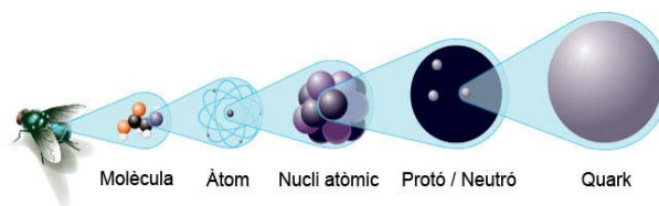
Figura 2. Els quarks són els constituents últims del nucli atòmic. Juntament amb els electrons formen els àtoms i els objectes. (Font: nobelprize.org ).
