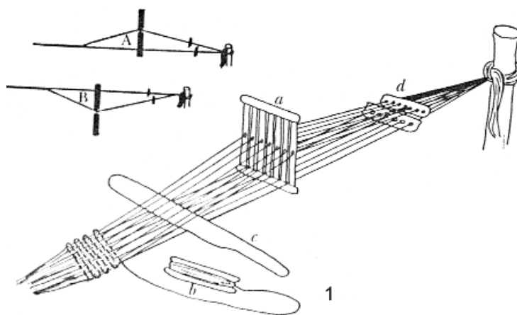
Fig. 5.1. Esquema de un telar de liza (según Alfaro 1997, fig. 16).
