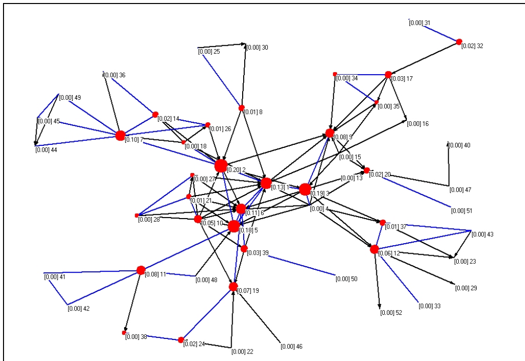
Figura 1. Valores de intermediación de la red primera
