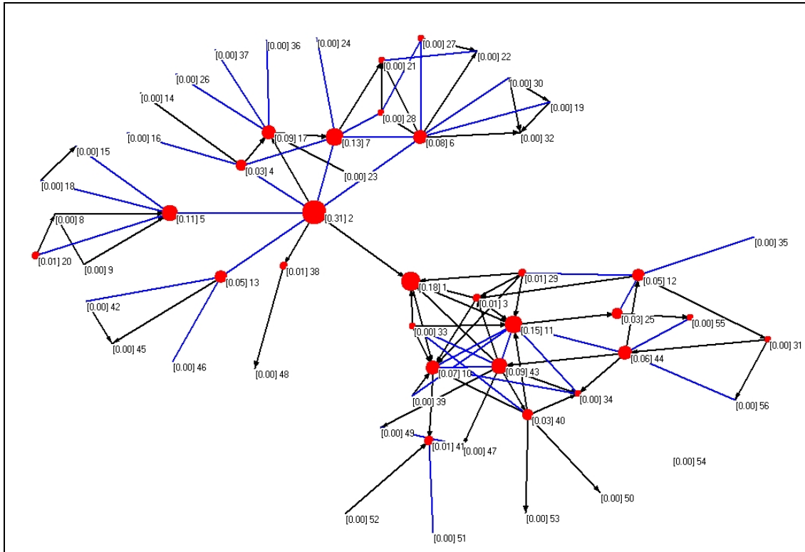
Figura 2. Valores de intermediación de la red segunda
